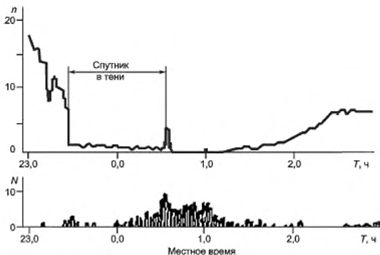
Рисунок В.8 — Связь частоты искрения с дифференциальной зарядкой
