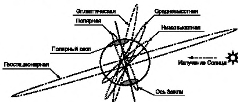
Рисунок В.1 — Типовые орбиты космических аппаратов
