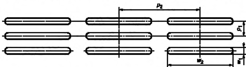
Рисунок В.1 — Щелевидные ячейки. Расположение рядами
