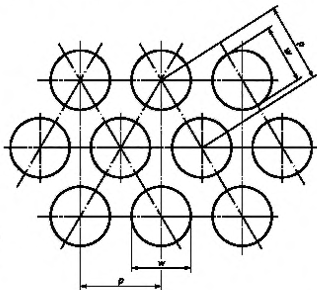
Рисунок А.1 — Круглые ячейки. Расположение в шахматном порядке
