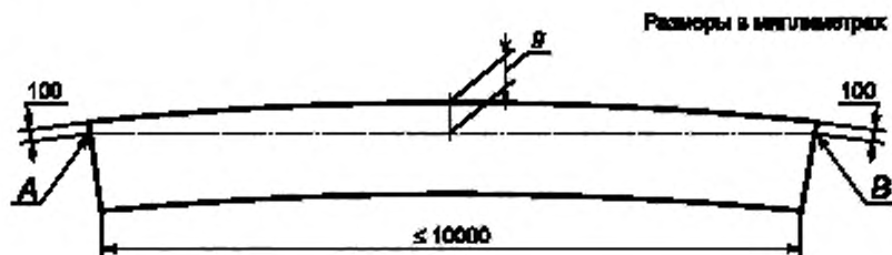
Рисунок 1 — Схема определения прямолинейности
