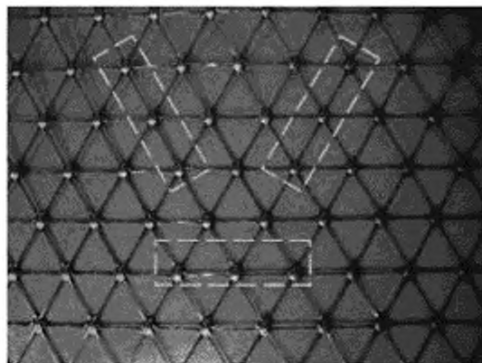
Рисунок А.2 — Схема отбора образцов для испытания на прочность ребра и прочность узла
