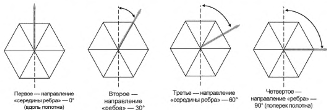
Рисунок А.1 — Четыре направления тестирования георешетки (два направления «середины ребра» и два направления «ребра»)
