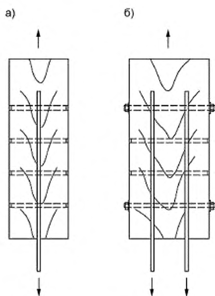
а — на нагелях; б — на нагелях и шпильках
