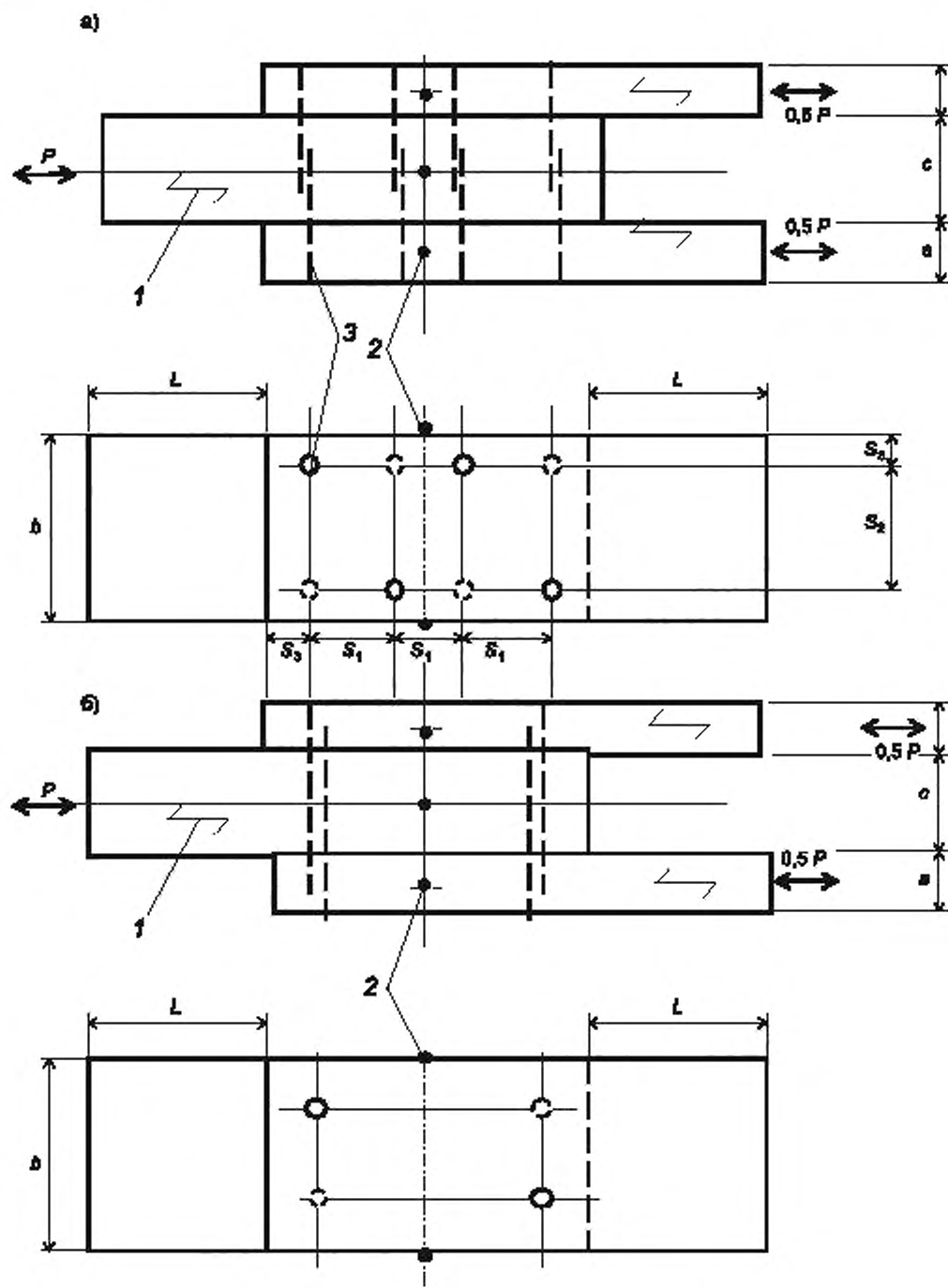
а — односрезных нагелей; б — двухсрезных нагелей 1 — направление волокон древесины; 2 — базовые точки для определения сдвига; 3 — нагели
