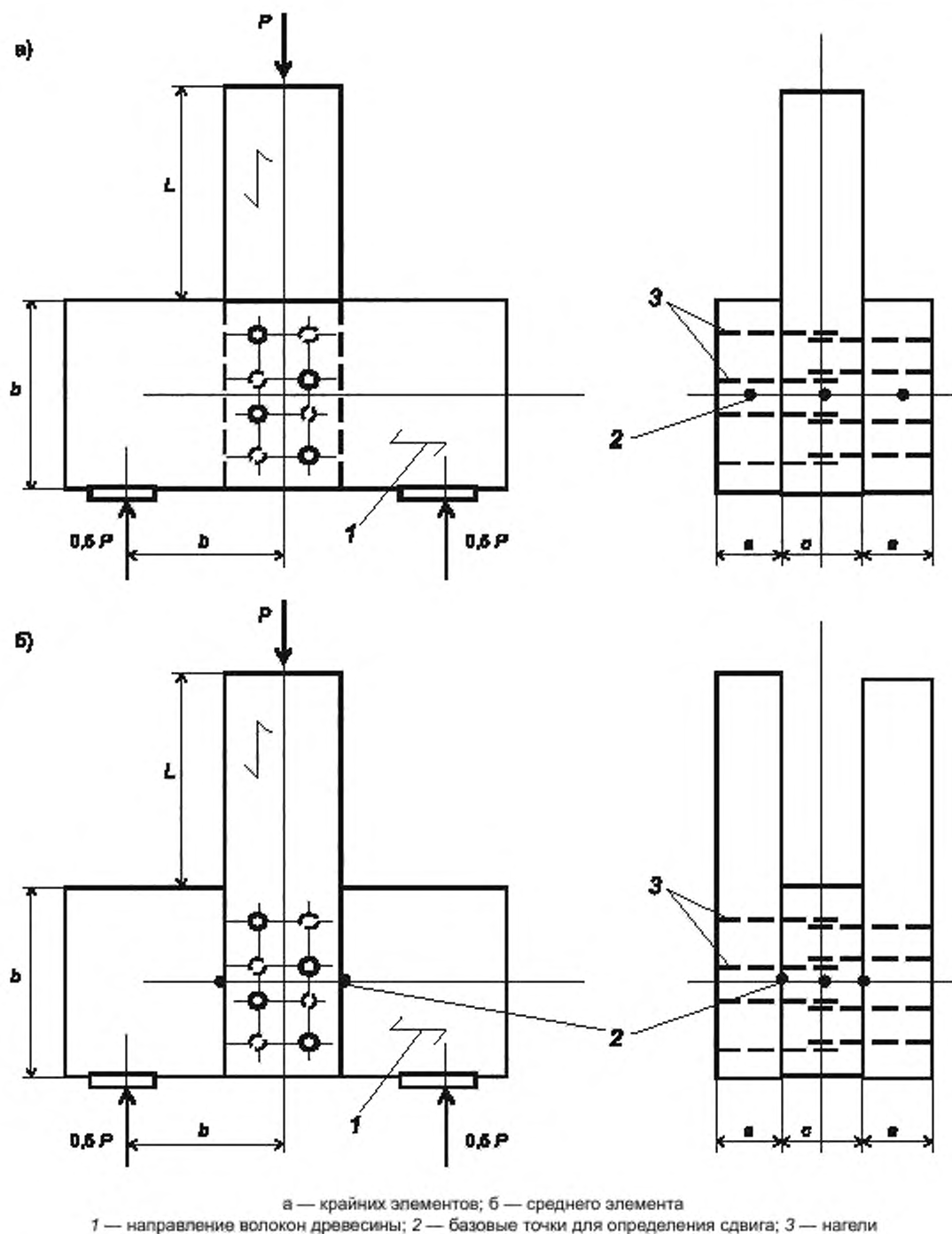
Рисунок 5 — Образец для испытания односрезных соединений при смятии поперек волокон древесины
