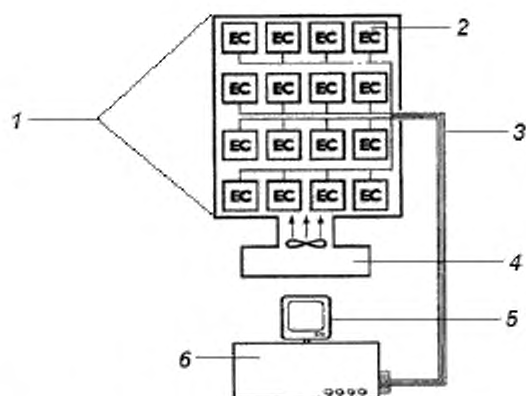
1 — плоскость испытания 1220 × 1830 мм; 2 — стекла с ЭХП; 3 — электрические выводы и кабели термодпар; 4 — термощаф; 5 — компьютер; 6 — многоканальная цифровая автоматизированная система управления и сбора данных
