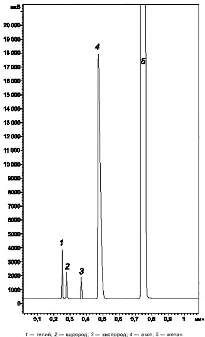
Рисунок Б.1 — Типовая хроматограмма гелия, водорода, кислорода, азота и метана в отпарном газе
