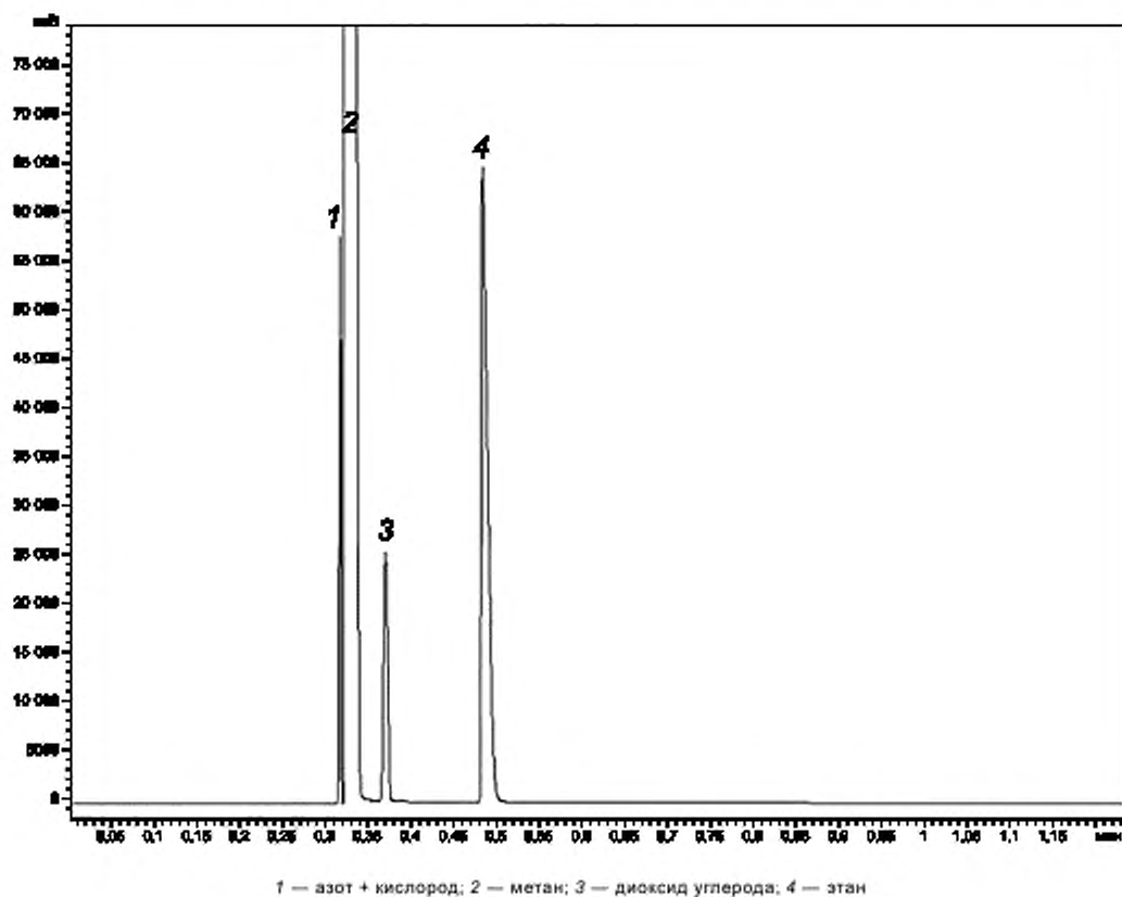
Рисунок А.1 — Типовая хроматограмма азота, метана, диоксида углерода и этана в отпарном газе
