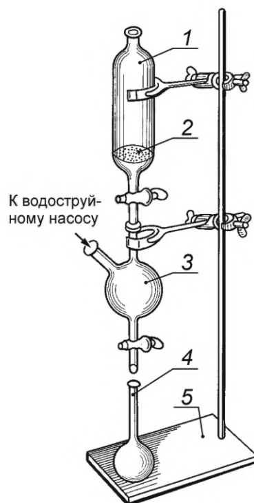
1 — фильтрующая делительная воронка; 2 — впаиванный стеклянный фильтр класса ПОР 100 или ПОР 160; 3 — приемник; 4 — мерная колба; 5 — штатив
