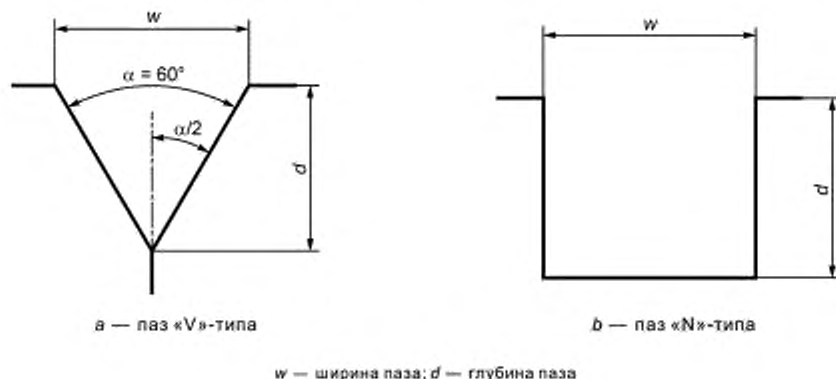
Рисунок 2 — Типы пазов «V» и «N»
