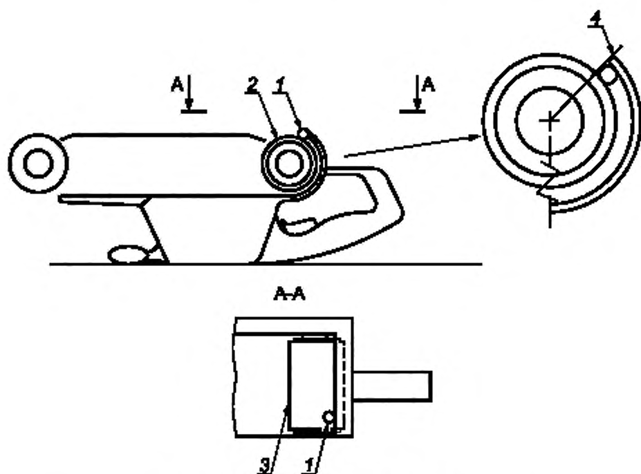
Рисунок 101 — Испытание стержневым щупом зазора между лентой и барабаном
