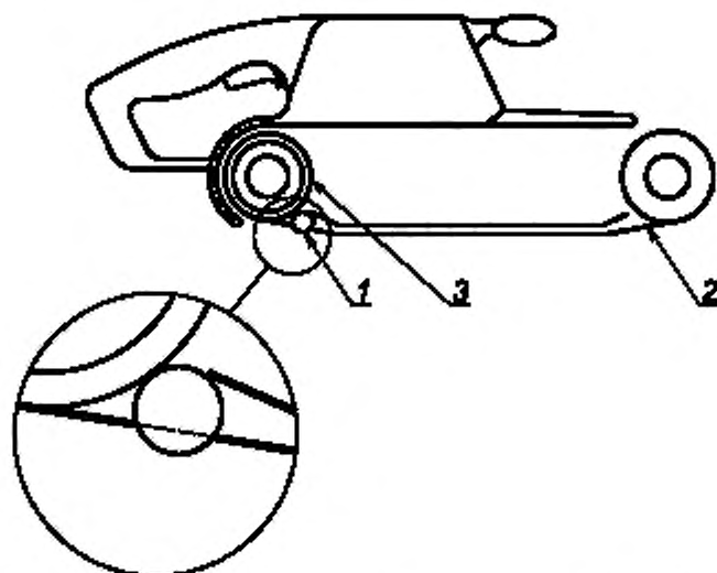
Рисунок 101 — Испытание стержневым щупом зазора между лентой и барабаном
