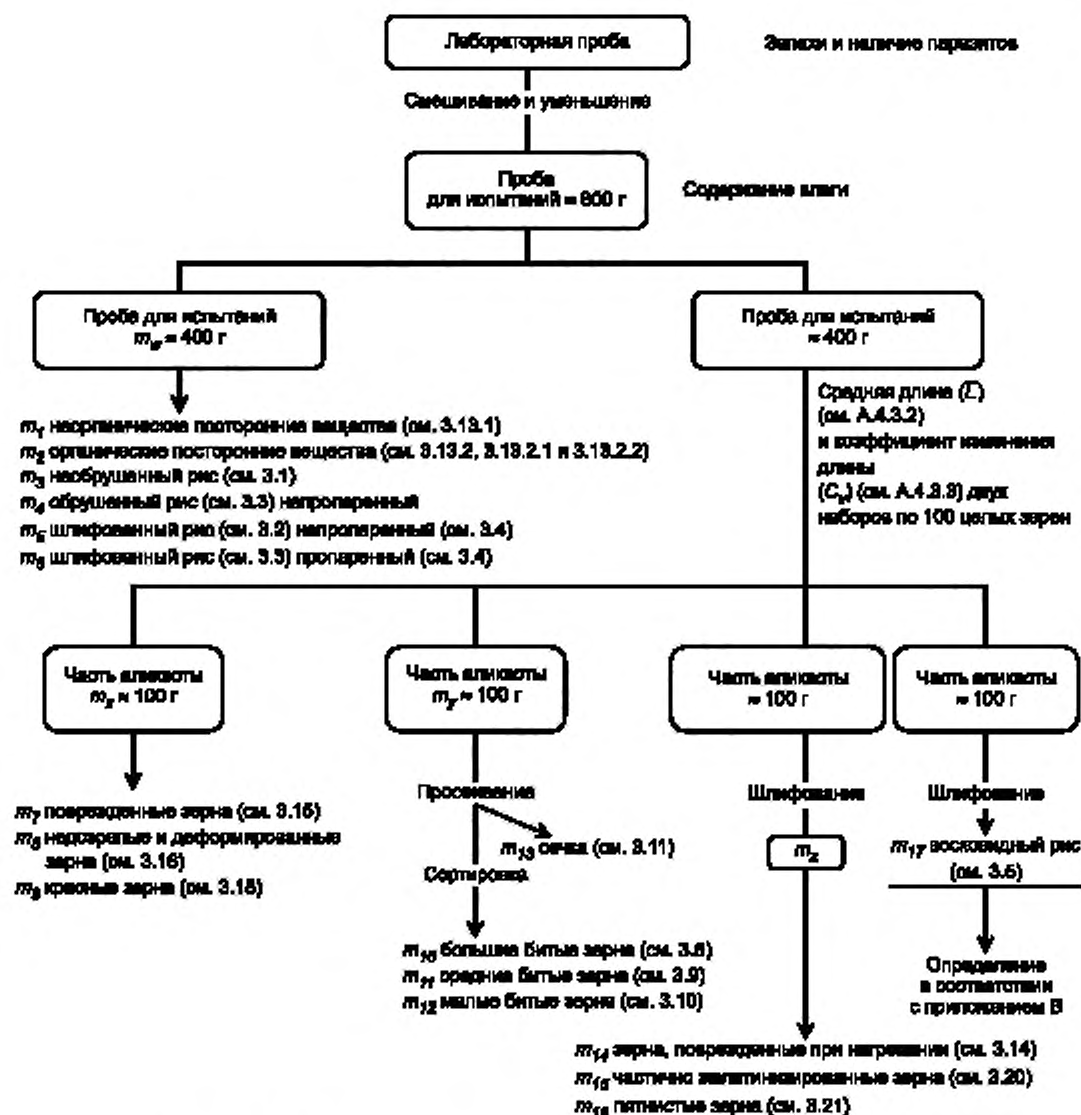
Рисунок А.3 — Схема определения категории зерна обрубленного риса пропаренного
