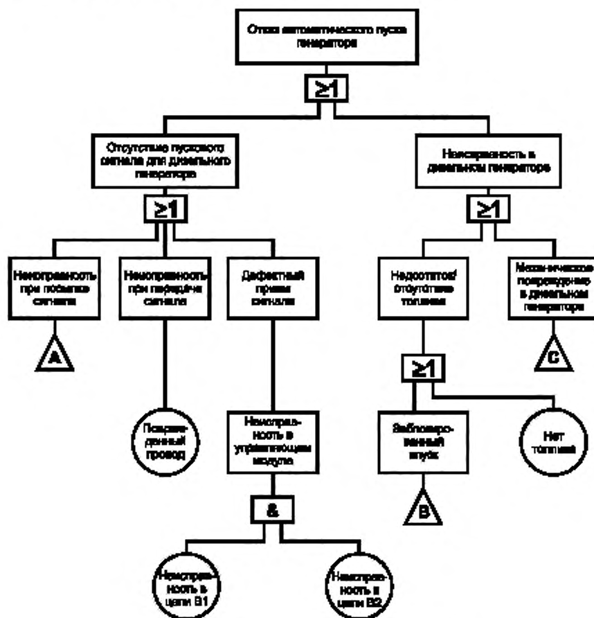
Рисунок А.1 — Пример «дерева неисправностей»
