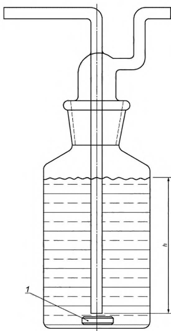
Рисунок 2 — Пример промывочного сосуда
