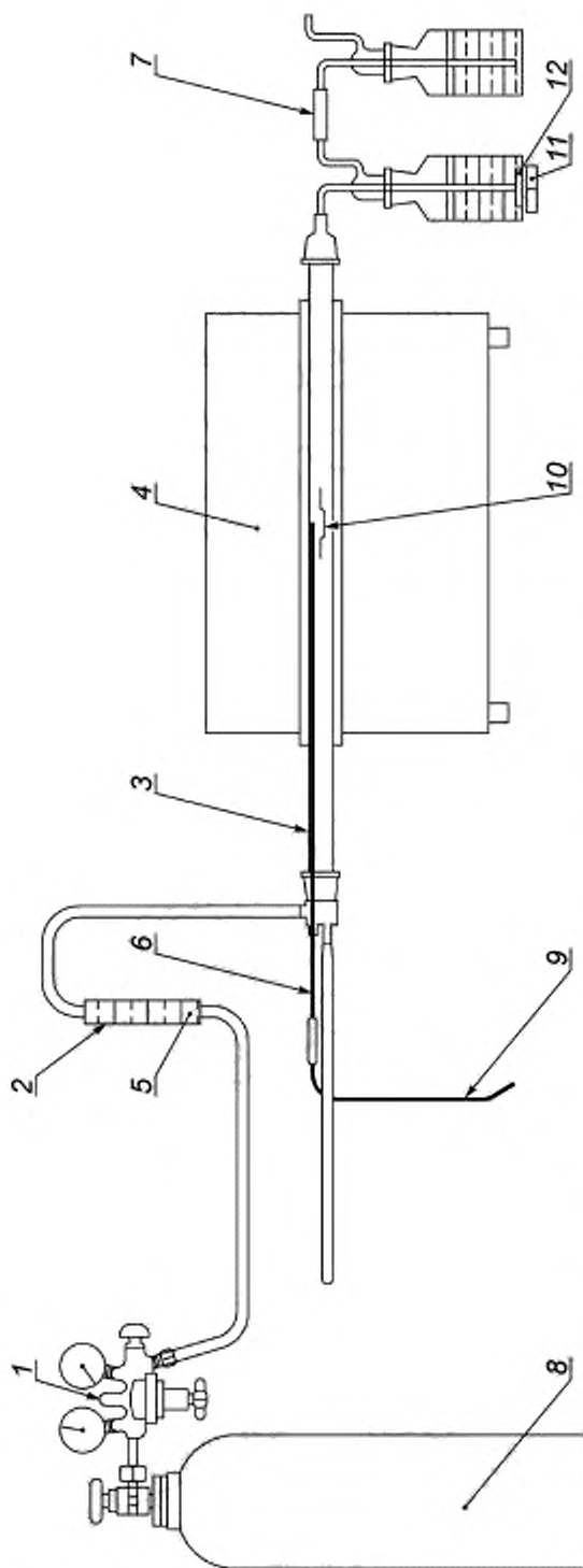
1 — редуктор, 2 — ротаметр, 3 — трубка из кварцевого стекла, 4 — печь, 5 — игольчатый вентиль, 6 — термолара, 7 — промывочные сосуды, 8 — искусственный воздух, 9 — устройство для ввода лодочки для сжигания с испытываемым образцом, 10 — лодочка для сжигания с испытываемым образцом, 11 — магнитная мешалка, 12 — стержень магнитной мешалки
