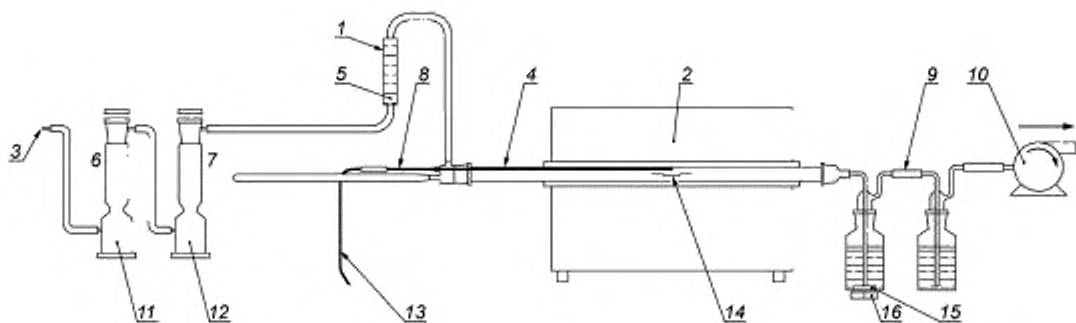
1 — редуктор; 2 — печь; 3 — воздух окружающей среды; 4 — трубка из кварцевого стекла; 5 — игольчатый вентиль; 6 — активированный уголь; 7 — силикагель; 8 — термометр; 9 — промывочные сосуды; 10 — всасывающий насос; 11 — воздушный фильтр; 12 — осушитель воздуха; 13 — устройство для ввода лодочки для сжигания с испытуемым образцом; 14 — лодочка для сжигания с испытуемым образцом; 15 — стержень магнитной мешалки; 16 — магнитная мешалка
