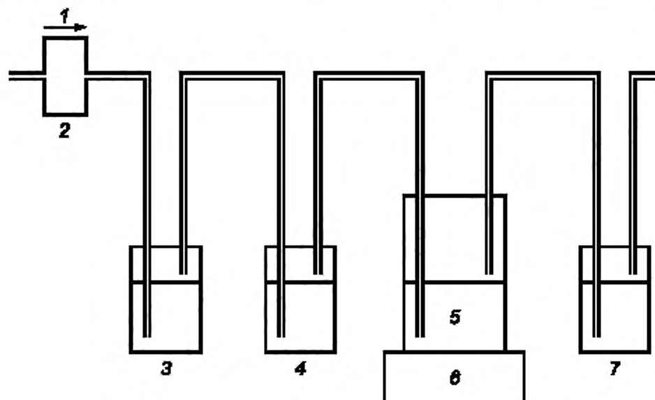
Рисунок А.1 — Принцип работы испытательной системы для измерения диоксида углерода
