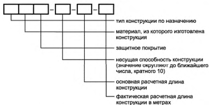
Рисунок А.1 — Условное обозначение ригелей
