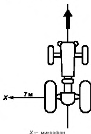
Рисунок 2 — Схема измерений внешнего шума неподвижного трактора
