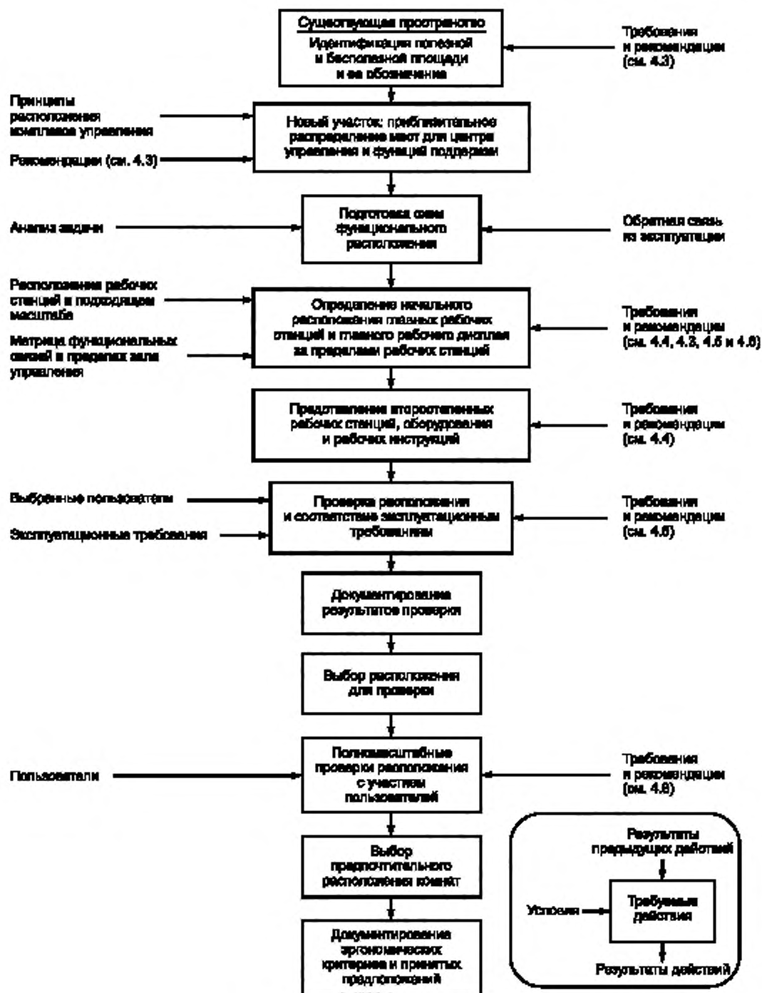
Рисунок 3 — Блок-схема процедуры планировки зала управления
