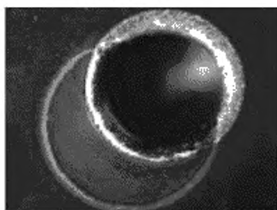
Погадание паяльной маски на монтажную контактную площадку
