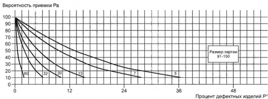
Рисунок С.5 — Объем партии от 51 до 90
