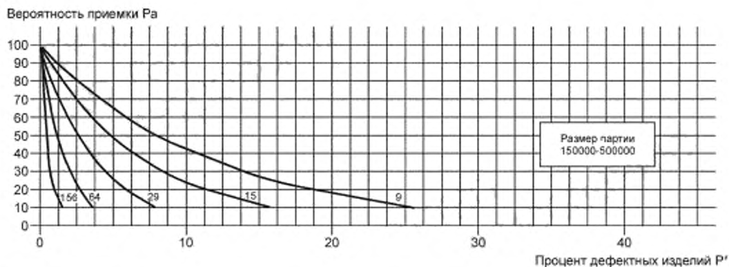
Рисунок С.13 — Объем партии от 35000 до 150000
