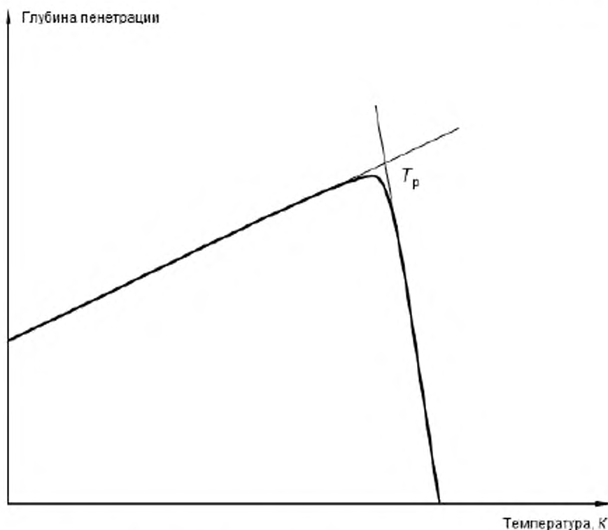
Рисунок 1 — Определение температуры пенетрации
