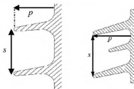
Постоянный вылет ребра
