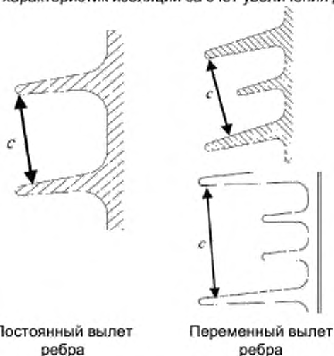
Рисунок 10 — Межреберное расстояние разных типов изоляторов
