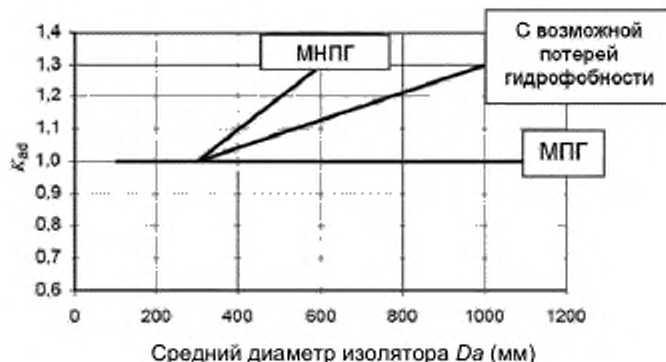
Рисунок 17б — K_{ад} в зависимости от среднего диаметра изолятора
