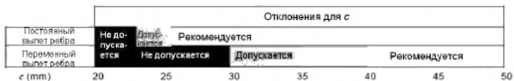
Рисунок 11 — Рекомендации по выбору межреберного расстояния
