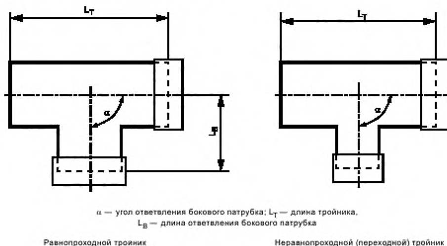
Рисунок 7 — Тройники
