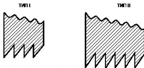
Рисунок 3 — Форма поперечного сечения уплотнительных колец муфт типа «REKA»
