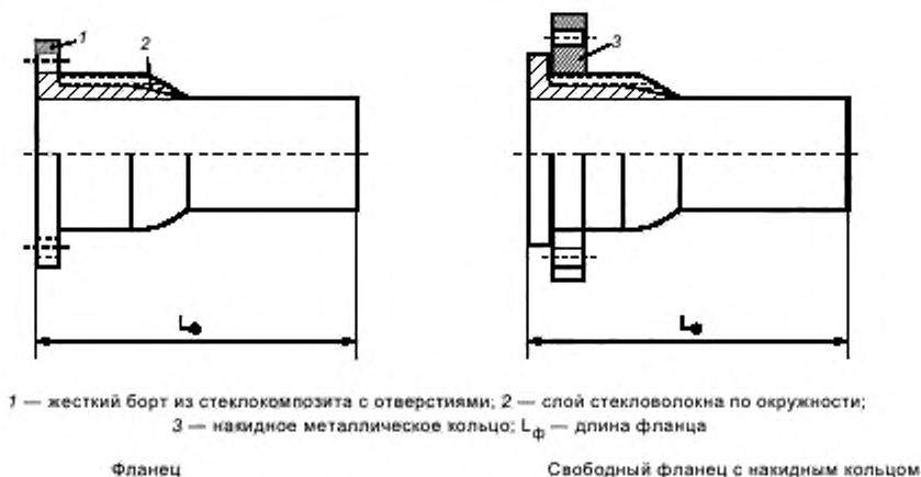
Рисунок 8 — Фланцы
