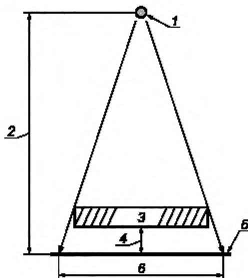
1 -- источник излучения; 2 -- расстояние от источника до детектора; 3 -- образец для контроля; 4 -- расстояние от образца для контроля до детектора; 5 -- детектор; 6 -- оптическое увеличение поля обзора
