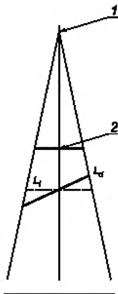
1 — источник излучения; 2 — образец для контроля; L_n — размер неискаженного изображения; L_d — размер искаженного изображения
