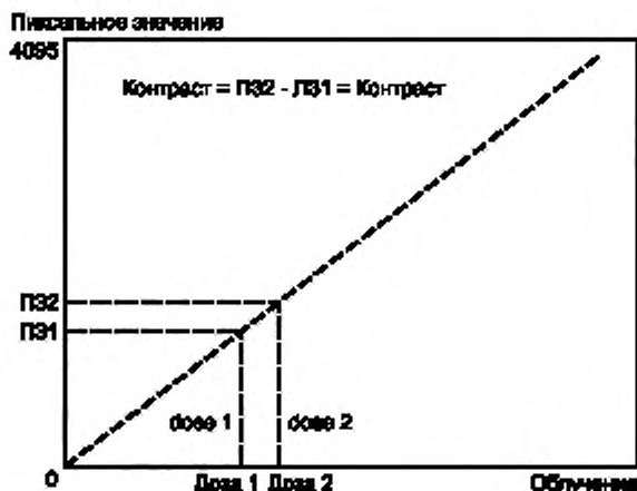
Рисунок ДЕ.3 — Зависимость облучения от пиксельного значения
