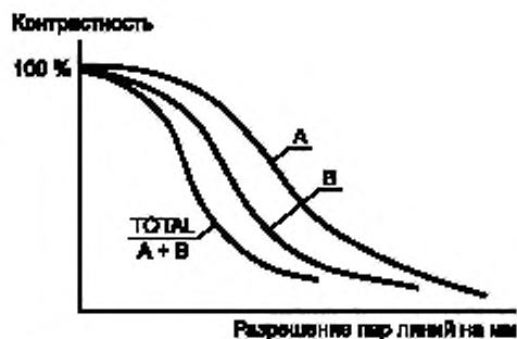
Рисунок ДГ.17 — Типичный график МТФ
