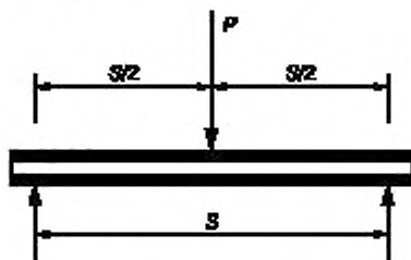
(a) трехточечное нагружение (C393/C393M стандартная схема)
