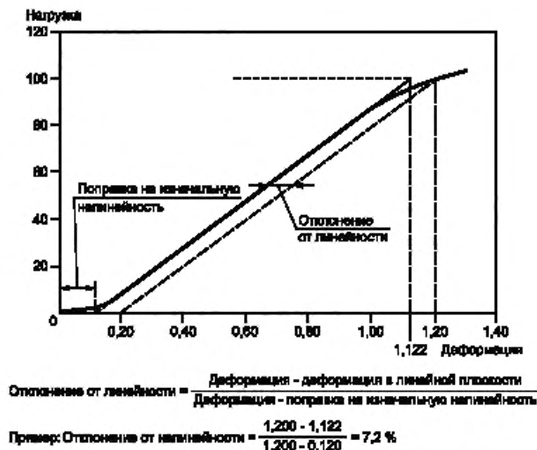
Рисунок 2 — Определение отклонения от линейности
