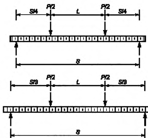
(c) четырехточечное нагружение (C393/C393M нестандартная схема)
