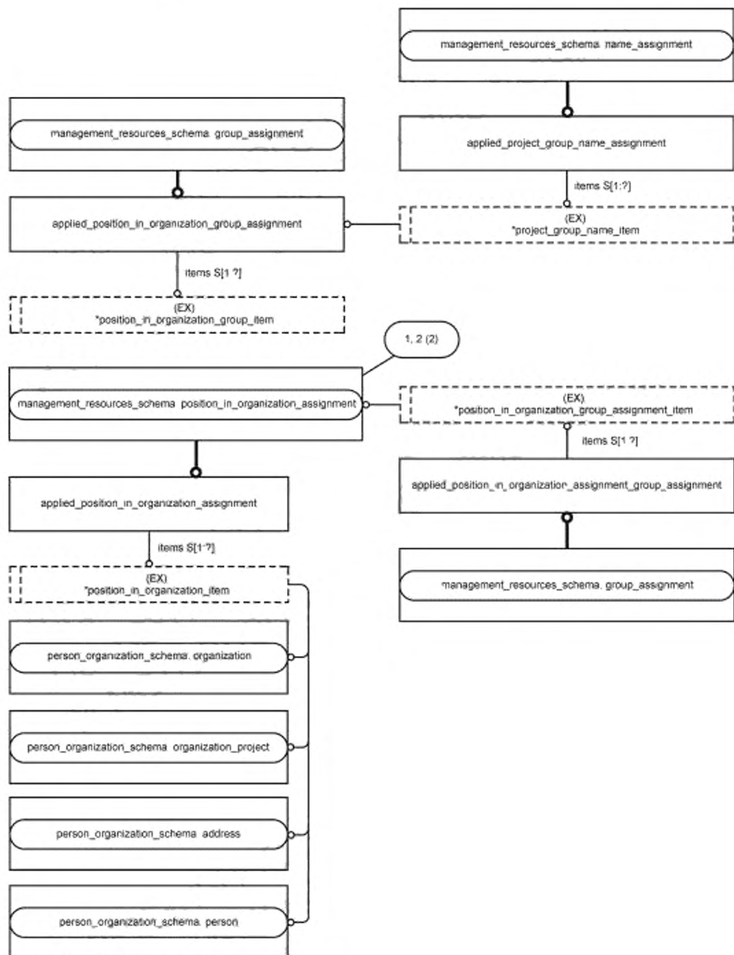
Рисунок D.2 — Представление IMM на уровне объектов в формате EXPRESS-G (диаграмма 1 из 2)
