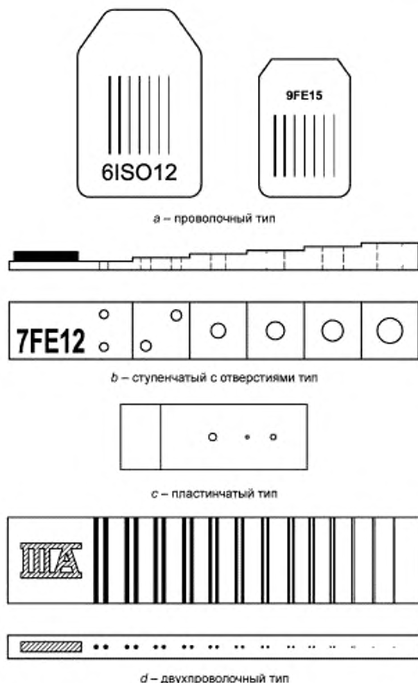
Рисунок 4 — Типы индикаторов качества изображения (IQI)
