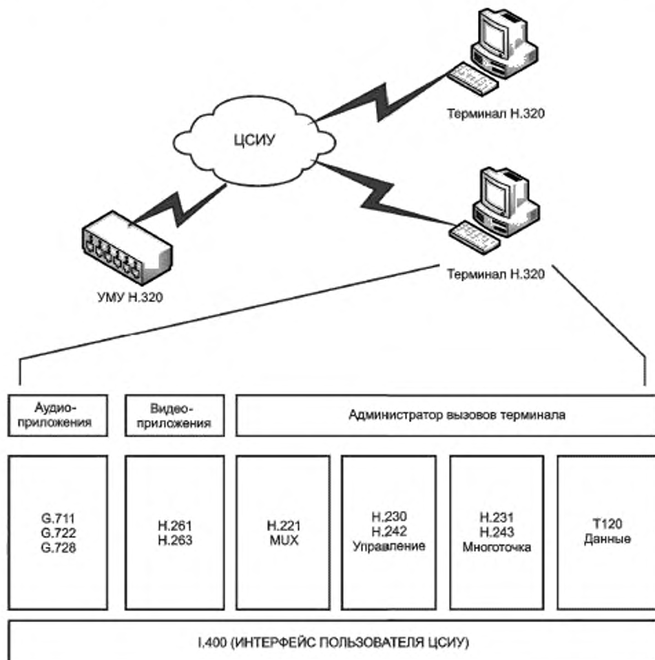
Рисунок 12 — Интероперабельность H.320
