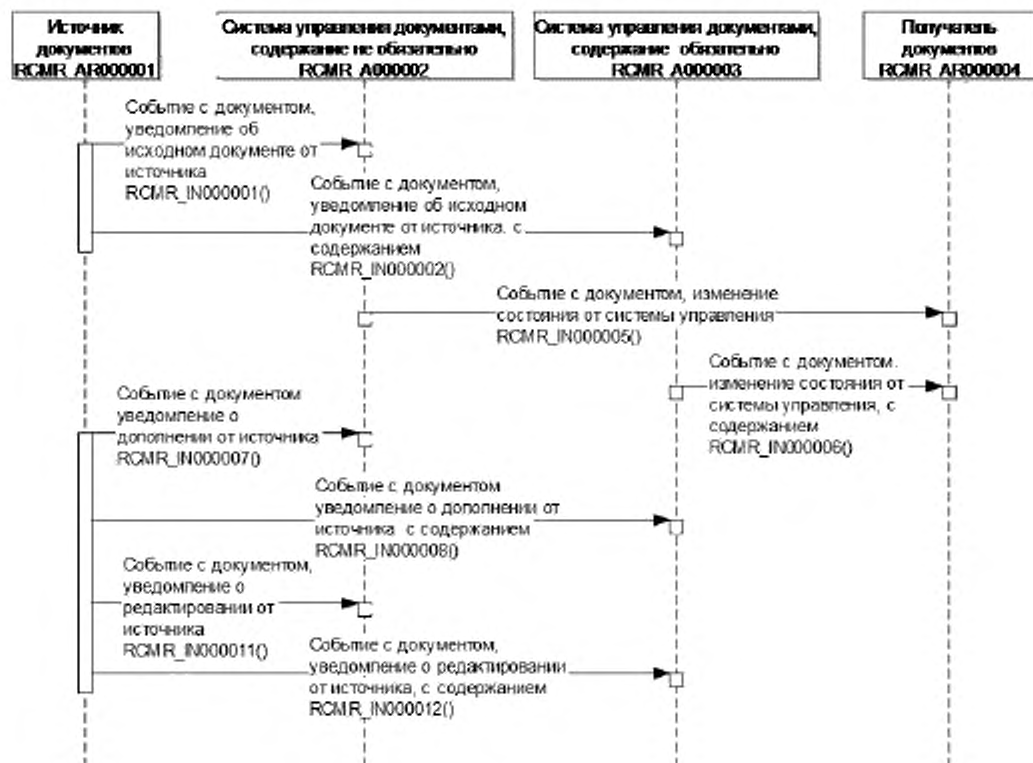
Рисунок G.10 — Пример диаграммы взаимодействия
