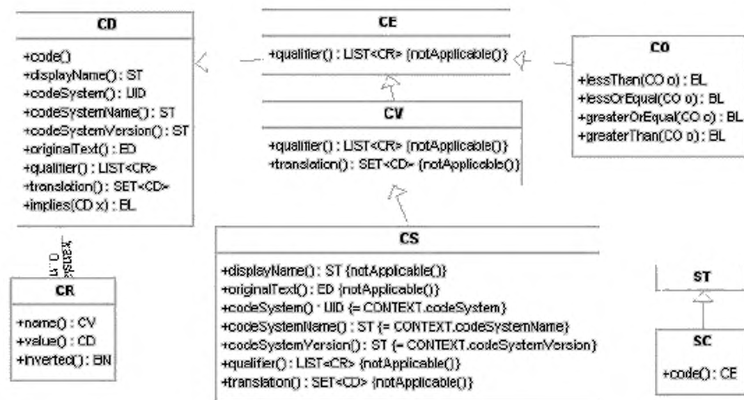
Рисунок В.4 — Информационная модель дескриптора понятия
