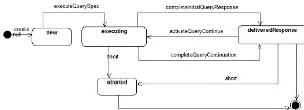
Рисунок A.14 — Диаграмма перехода состояний класса QueryEvent (событие запроса)
