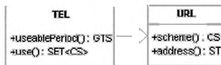
Рисунок В.7 — Типы данных URL и TEL
