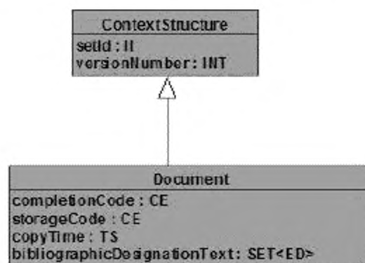
Рисунок A.9 — Диаграмма классов предметной области StructuredDocuments (структурированные документы)
