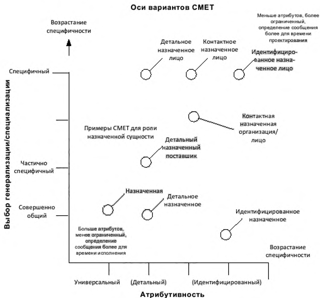
Рисунок G.4 — Варианты СМЕТ
