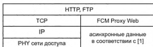
Рисунок 11 — Структура процесса преобразования протоколов сети доступа IP туннелированием внутри транспортного протокола HLN
