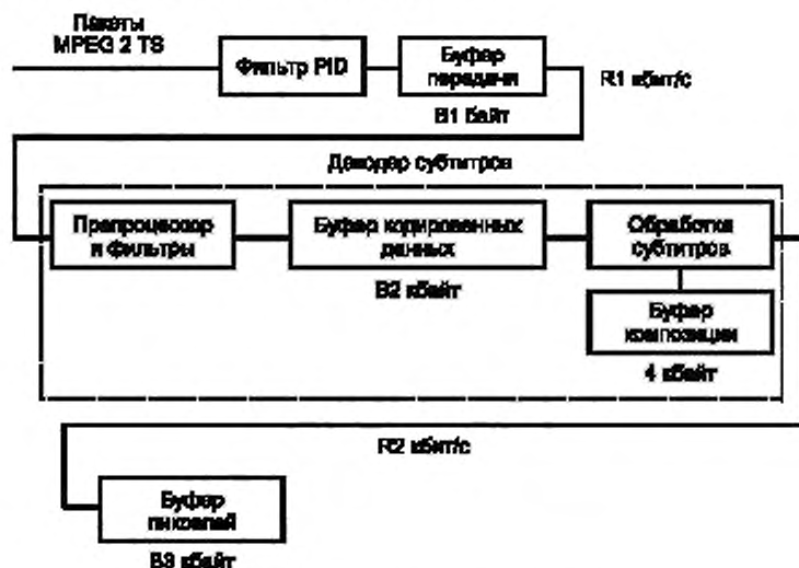
Рисунок 2 — Модель декодера субтитров
