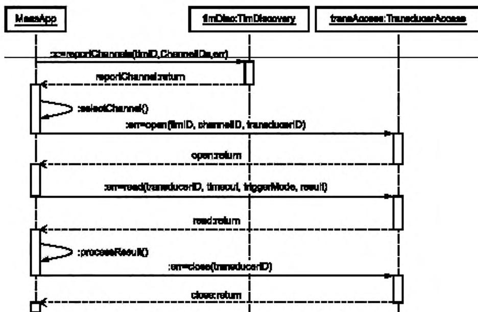
Рисунок В.1 — Простой пример «опрошенного» измерения
