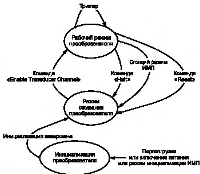
Рисунок 3 — Режимы работы канала преобразователя
