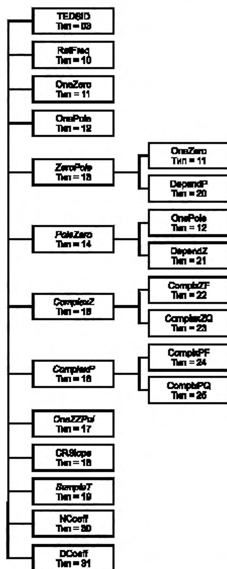
Рисунок 19 — Структура ЭТДП передаточной функции
