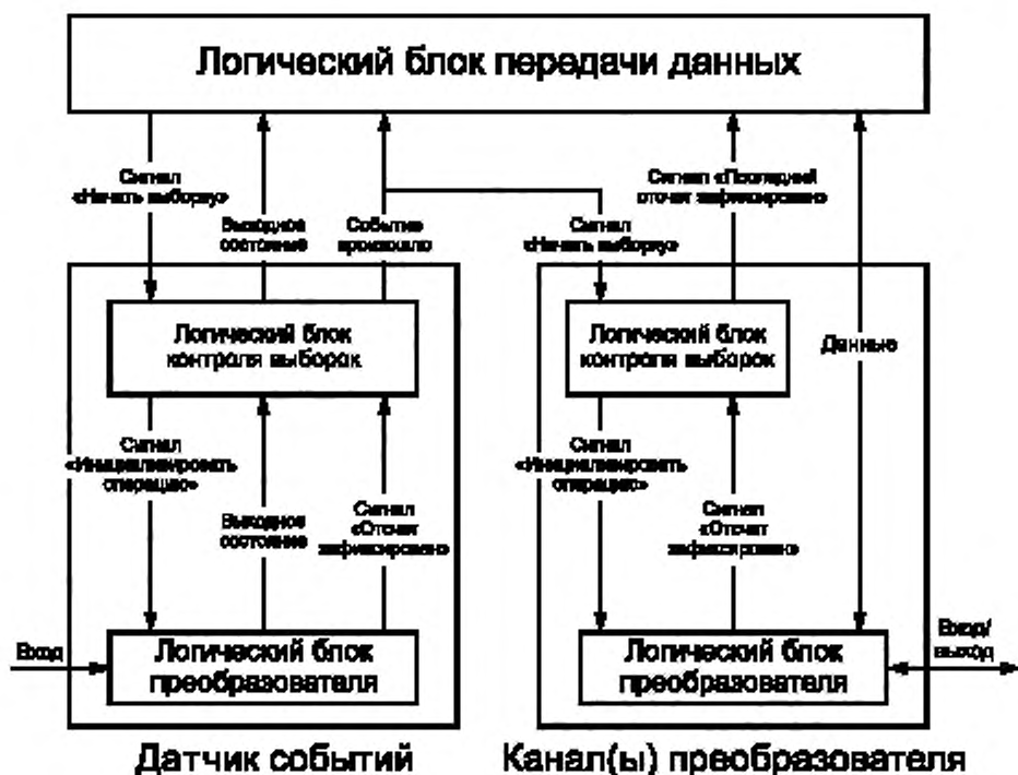
Рисунок 10 — Выход датчика событий, использующийся в качестве триггера
