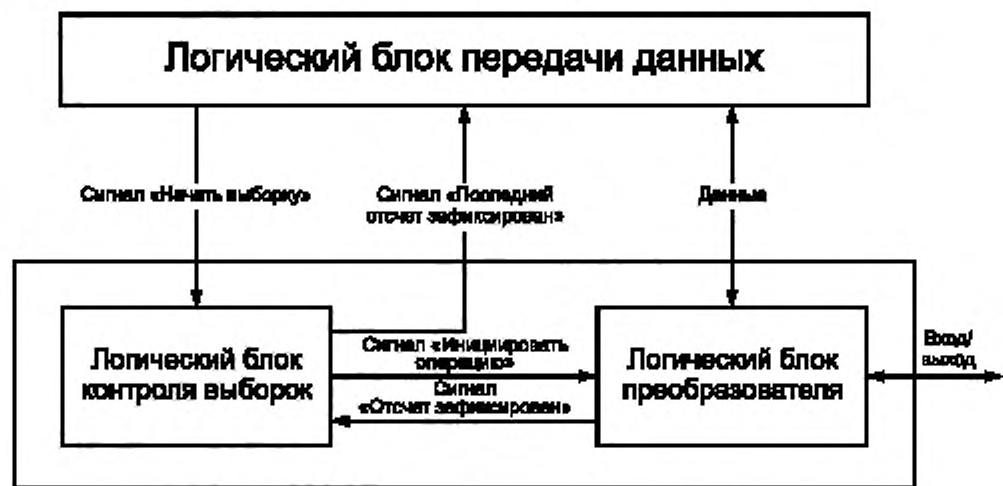
Рисунок 9 — Элементарные функциональные блоки канала преобразователя
