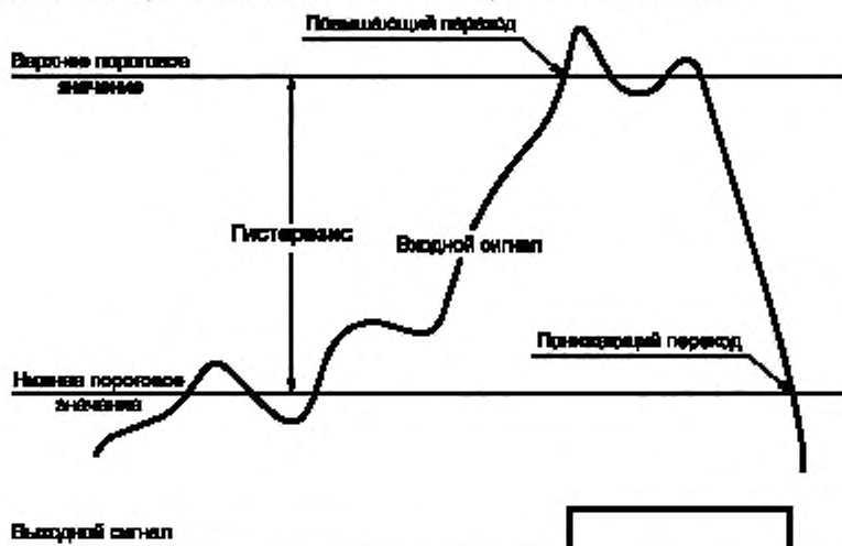
Рисунок 5 — Характеристика аналогового датчика событий
