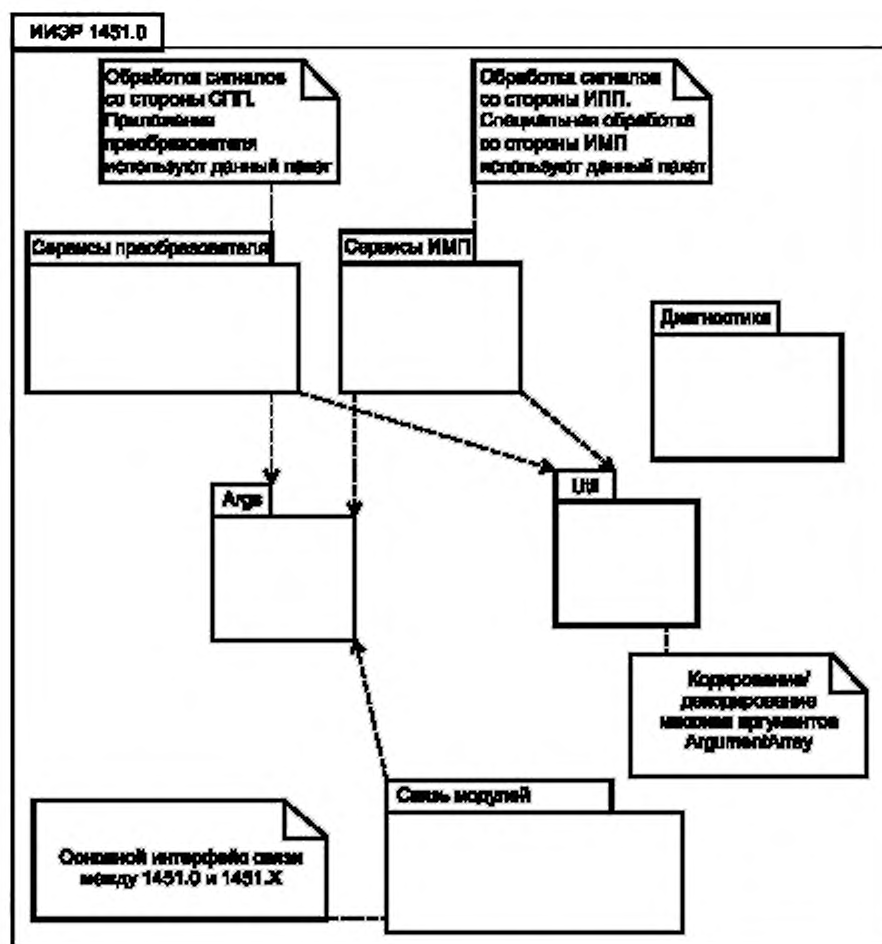
Рисунок 21 — Структура API
