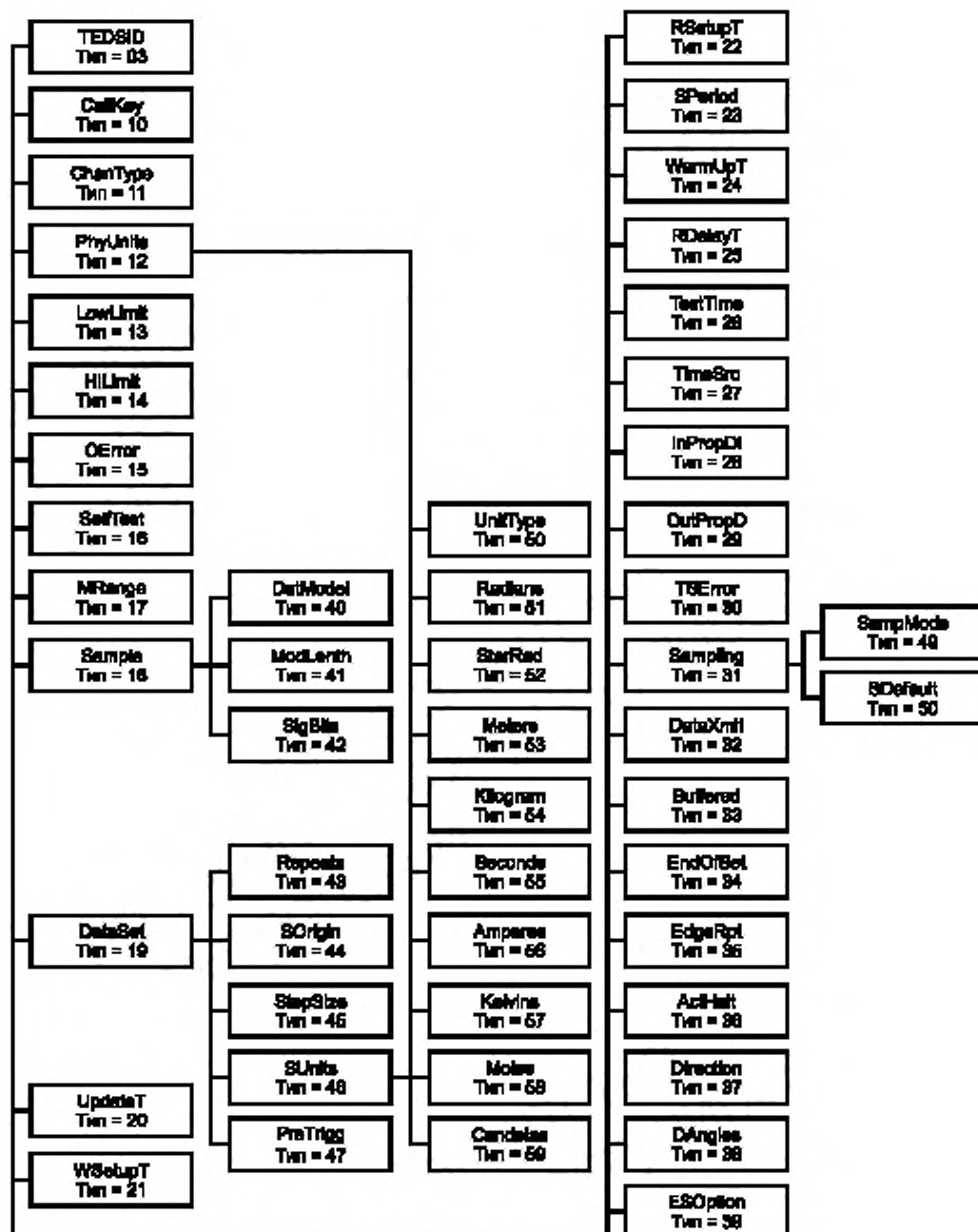
Рисунок 14 — ЭТДП канала преобразователя
