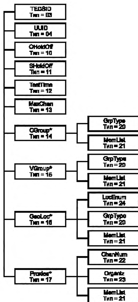
Рисунок 13 — Структура блока данных мета-ЭТДП
