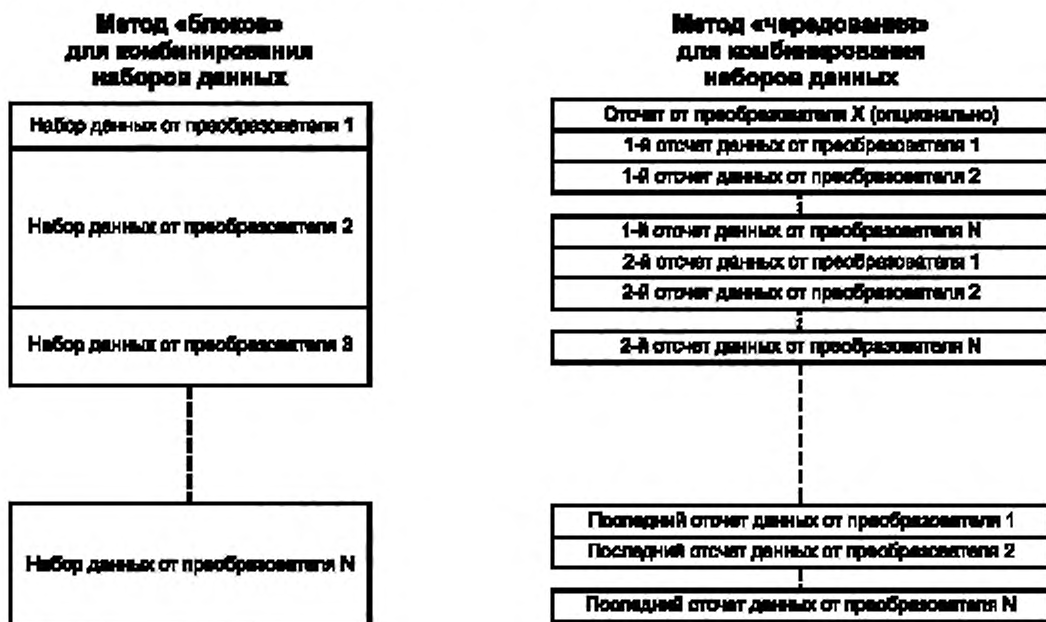
Рисунок 6 — Методы комбинирования наборов данных
