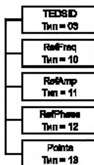
Рисунок 18 — Структура ЭТДП частотной характеристики
