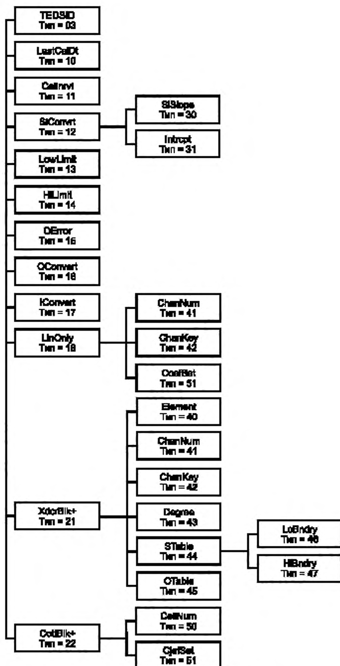
Рисунок 16 — Структура ЭТДП калибровки
