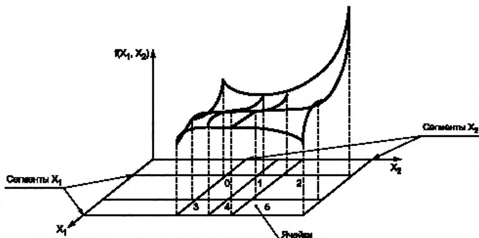
Рисунок 15 — Двумерная функция, разбитая на ячейки 2x3
