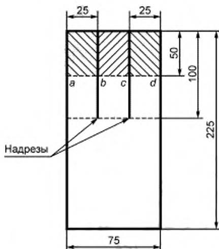
Рисунок 1 — Образец с тремя язычками
