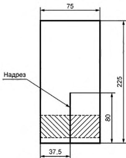
Рисунок 2 — Образец с двумя язычками
