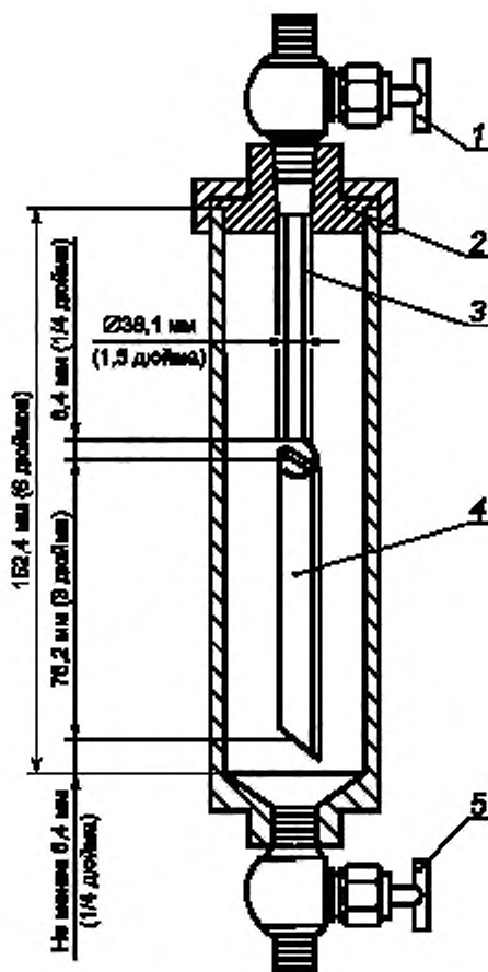
1 — игольчатый вентиль А диаметром 6,4 мм (1/4 дюйма); 2 — неопреновое уплотнительное кольцо; 3 — выпускная трубка; 4 — медная пластинка; 5 — игольчатый вентиль В диаметром 6,4 мм (1/4 дюйма)
