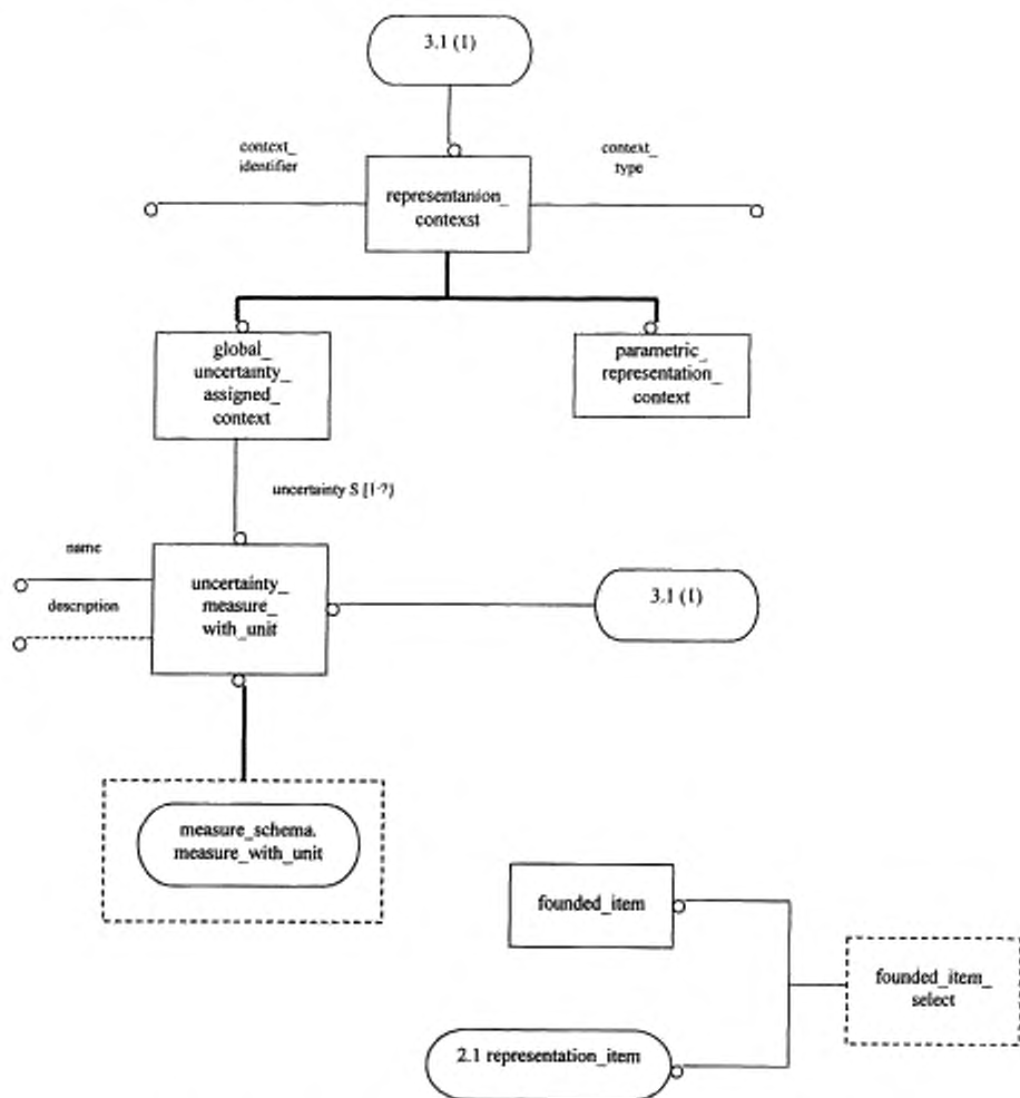
Рисунок D.3 — EXPRESS-G диаграмма representation_schema 3 из 3
