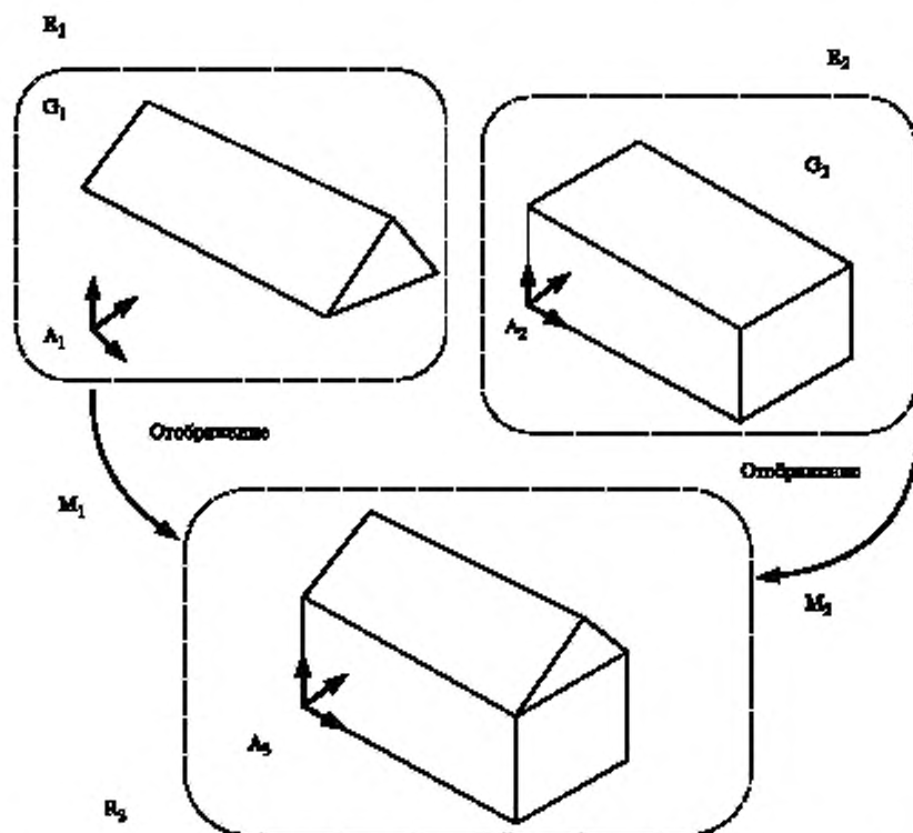
Рисунок 2 — Пример использования объектов mapped_item и representation_map
