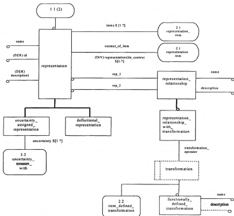
Рисунок D.1 — EXPRESS-G диаграмма representation_schema I из 3
