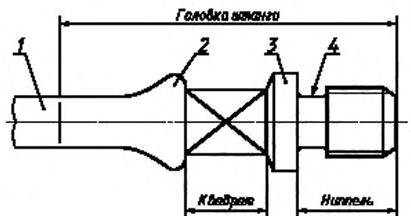
1 — тело штанги; 2 — подзеваторный бурт; 3 — упорный бурт; 4 — зарезбованная канавка
