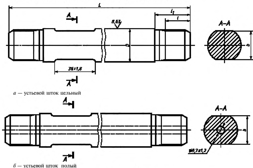
Рисунок 6 — Устьевой шток
