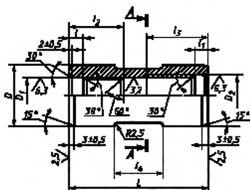
Рисунок 5 — Переводные муфты
