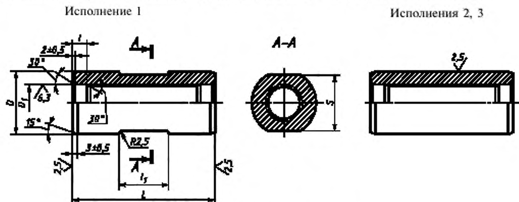
Рисунок 4 — Соединительные муфты
