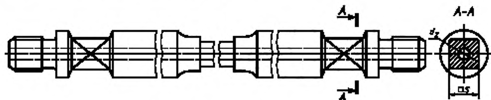
д — стеклопластиковая полая штанга (ШНСП)
