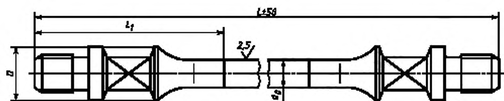
б — металлическая штанга с приваренными головками (ШНП)
