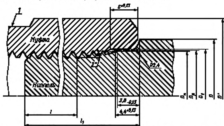
1 — поверхность под ключ; D_n — диаметр пояса ниппеля; D_p — диаметр расчетный теоретический; D_1 — диаметр выточки муфты; D — наружный диаметр устьевого штока; D' — наружный диаметр муфты; l — длина цилиндрической части резьбы ниппеля; l_2 — длина ниппеля
