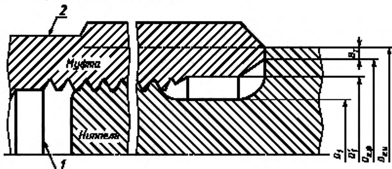
1 — плоскость конца резьбы муфты (продолжение резьбы муфты по выбору изготовителя); 2 — поверхность под ключ; B_1 — ширина торцевой контактной поверхности; D_1 — диаметр зарезьбовой канавки ниппеля; D_1 — диаметр выточки муфты; D_{кв} — максимальный диаметр внутренней фаски муфты; D_{кв} — допускаемый минимальный диаметр изношенной муфты
