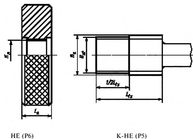
Рисунок Д.2 — Основные размеры калибров HE (P6) и К-HE (P5) для контроля резьбы ниппеля
