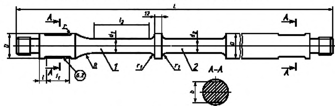
Рисунок 8 — Утяжеленная штанга
