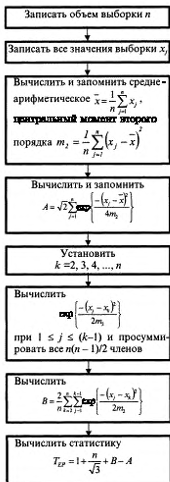
Рисунок 8 — Алгоритм вычисления статистики критерия Эппса-Палли T_{EP}
