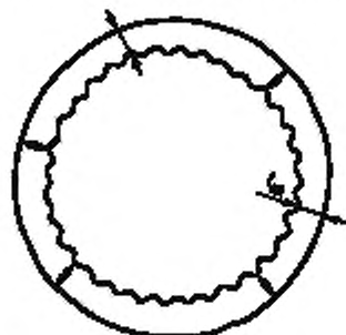
Рисунок 2 — Измерение толщины оболочки (круглый внутренний профиль неправильной формы)
