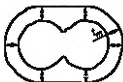
t_m — минимальная толщина
