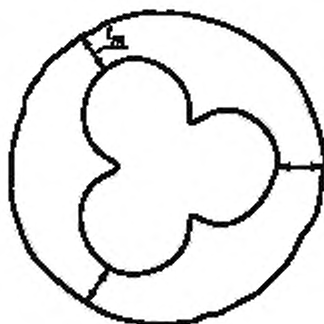
Рисунок 3 — Измерение толщины оболочки (некруглый внутренний профиль)
