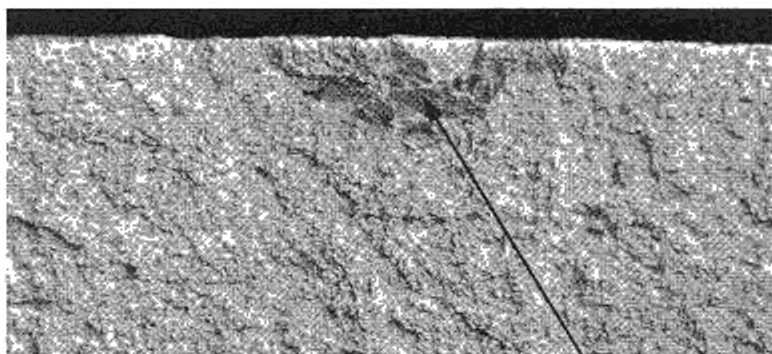
Макроструктура поперечного сечения прутка
