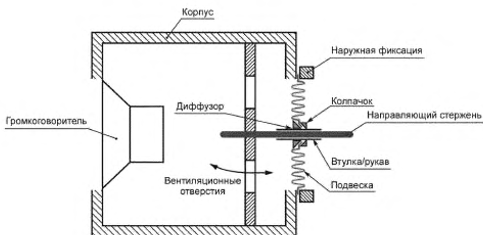
Рисунок 3 — Пневматическое возбуждение подвесной части
