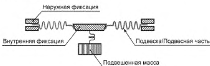
Рисунок 1 — Измерение статического смещения
