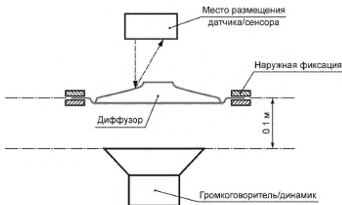
Рисунок 2 — Измерение наименьшей резонансной частоты f_0
