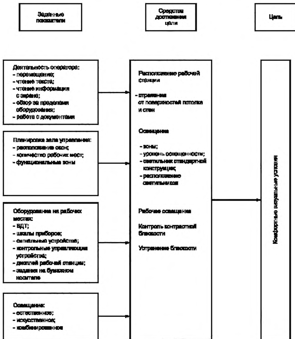
Рисунок 3 — Основные факторы при проектировании освещения центра управления
