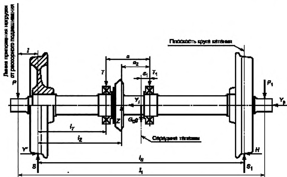
Рисунок А.3 — Схема действия нагрузок на КП с осевым редуктором
