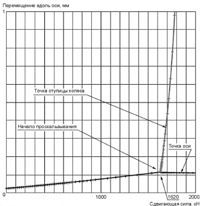
Рисунок Е.2 — Изменение перемещений точек ступицы колеса и оси в зависимости от сдвигающей силы
