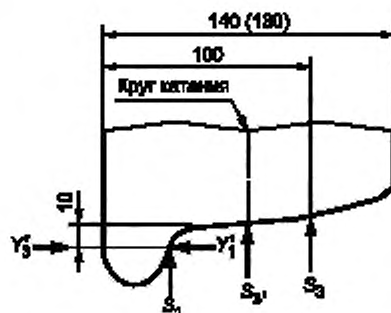
S, Y — вертикальная и боковая нагрузки на набегающее колесо от рельса при режимах: S_1 — движение по кривым участкам пути; S_2, S_3 — движение высокоскоростного ПС по специальному пути, S_3 — движение по стрелкам
