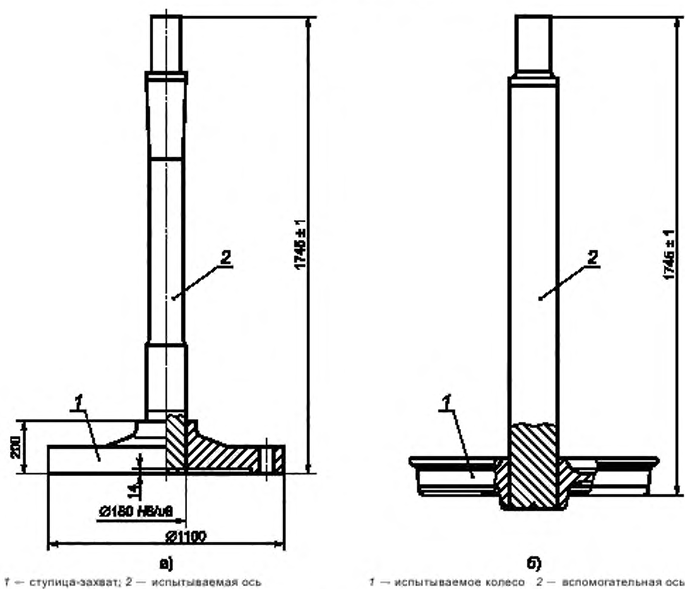
Рисунок И.1 — Образцы сборок для испытаний на усталость полномасштабных осей и колес
