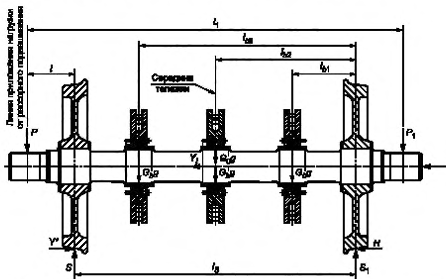
Рисунки А.3 и А.4 T(T_1) — вертикальная сила от опорно-осевого подшипника; P(P_1) — вертикальная нагрузка на буксовую шейку оси со стороны набегающего (сбегающего) колеса; S(S_1) — вертикальная нагрузка на набегающее (сбегающее) колеса от рельса; Z — вертикальная сила на ось от ведомой шестерни; H — поперечная составляющая силы трения внутреннего колеса о рельс; Y — боковая сила рельса на набегающее колесо; Y_1 — поперечная сила инерции КП; Y_0 — рамная сила; l_1 — расстояние между линиями приложения вертикальной нагрузки к буксовым шейкам оси колесной пары; l_2 — расстояние между плоскостями кругов катания КП; l_3 — расстояние от плоскости круга катания набегающего колеса до линии действия силы T ; l_4 — расстояние от плоскости круга катания набегающего колеса до линии действия силы Z ; G_0 — масса части оси, заключенной между плоскостями кругов катания колес; G_b — масса дискового тормоза; g — ускорение силы тяжести; a — расстояние между силами T и T_1 ; a_1 — расстояние от середины тележки до силы T_1 ; a_2 — расстояние между силами T и Z ; l_{b1} , l_{b2} , l_{b3} — расстояния от центра тяжести дисковых тормозов до сбегающего колеса
