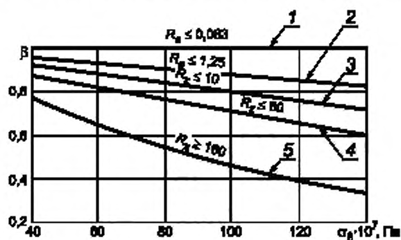
Рисунок 5 — Влияние состояния поверхности на предел выносливости
