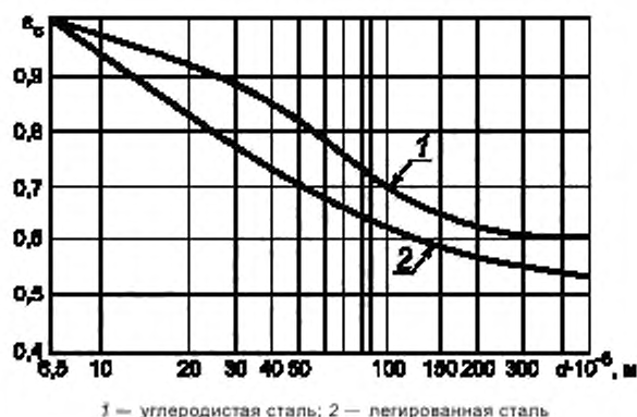
Рисунок 4 — Коэффициенты влияния абсолютных размеров сечения \epsilon_{\sigma} на усталостную прочность \beta — коэффициент влияния на предел выносливости качества обработки поверхности (рисунок 5);
