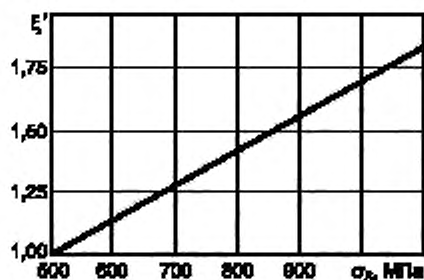
Рисунок 7 — Поправочные коэффициенты \xi' и \xi''
