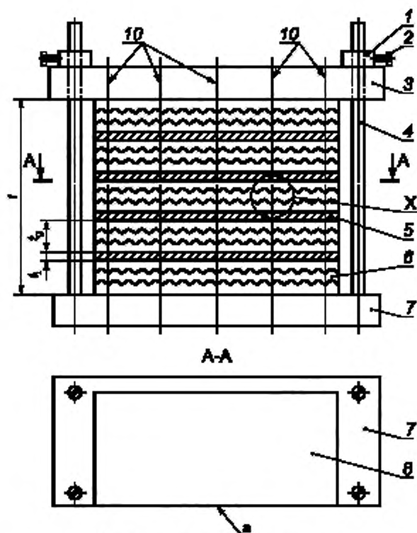
Рисунок 1 — Пример прибора для определения толщины одиночных слоев многослойных изделий
