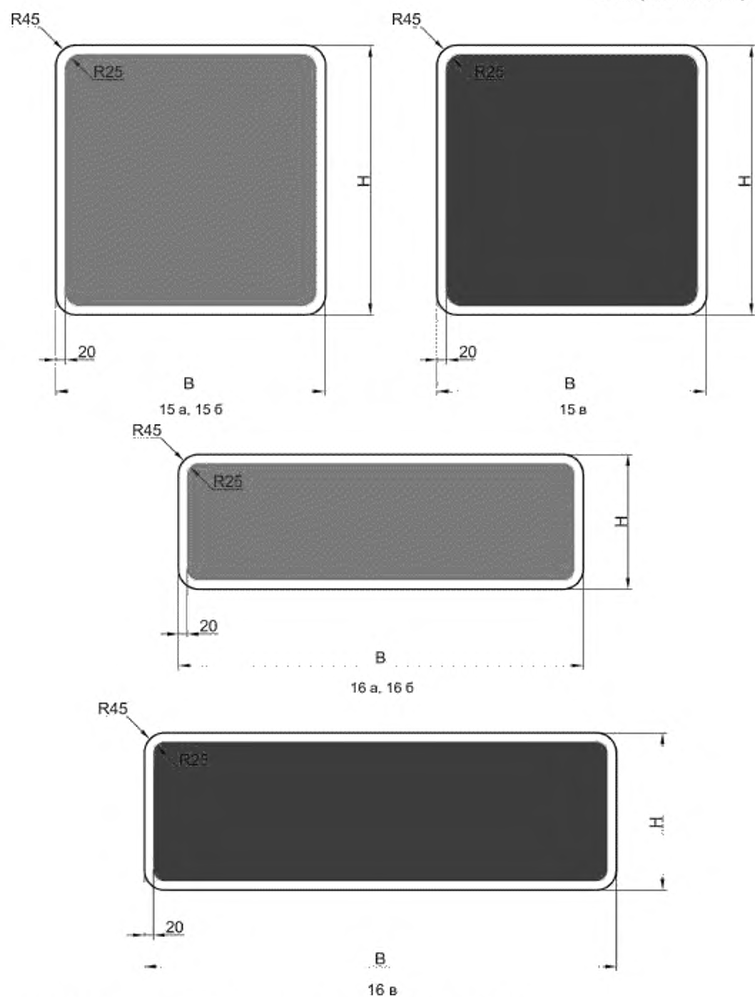
Рисунок А.1, лист 5
