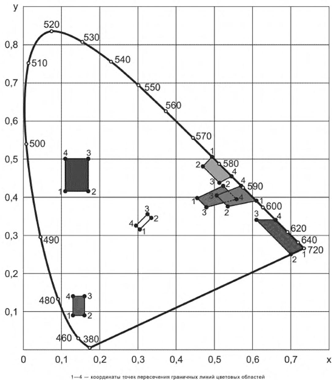
Рисунок Е.4 — График цветных областей изображений дорожных знаков (световозвращающий материал II класса с высокой цветоустойчивостью и световозвращающий материал III класса без свойств флуоресценции)
