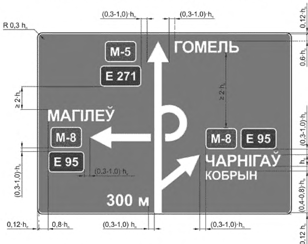
Рисунок В.1 — Пример компоновки изображения знака вида 27
