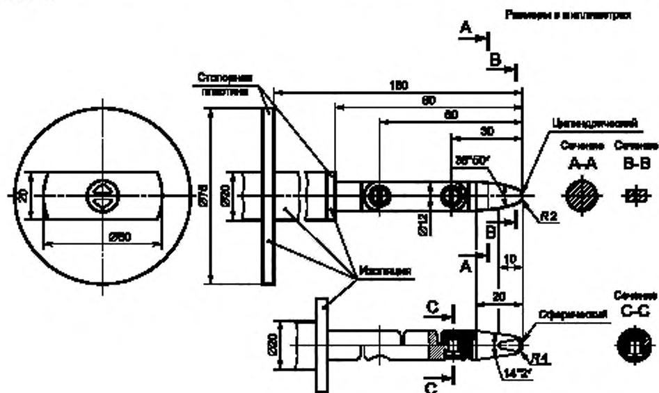
Рисунок 2 — Шарнирный шуп
