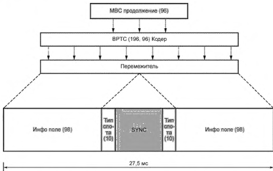
Рисунок А.27 — Формат пакета промежуточного MBC сообщения
