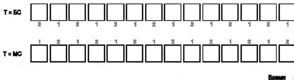
Рисунок А.13 — Диаграмма выровненной синхронизации канала
