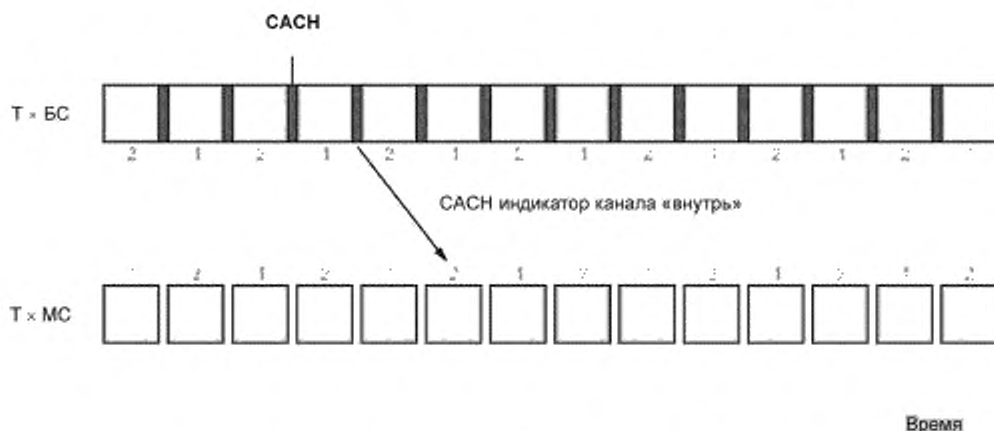
Рисунок А.7 — Синхронизация между пакетами CACH и «внутри»
