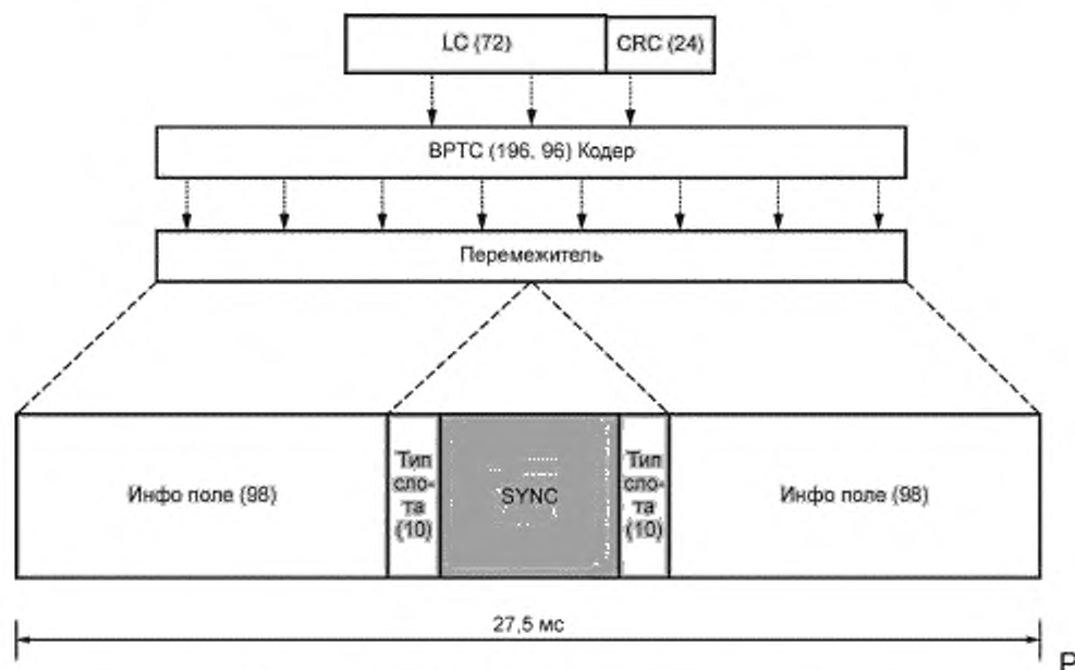
Рисунок А.22 — Формат LC пакета голосового заголовка
