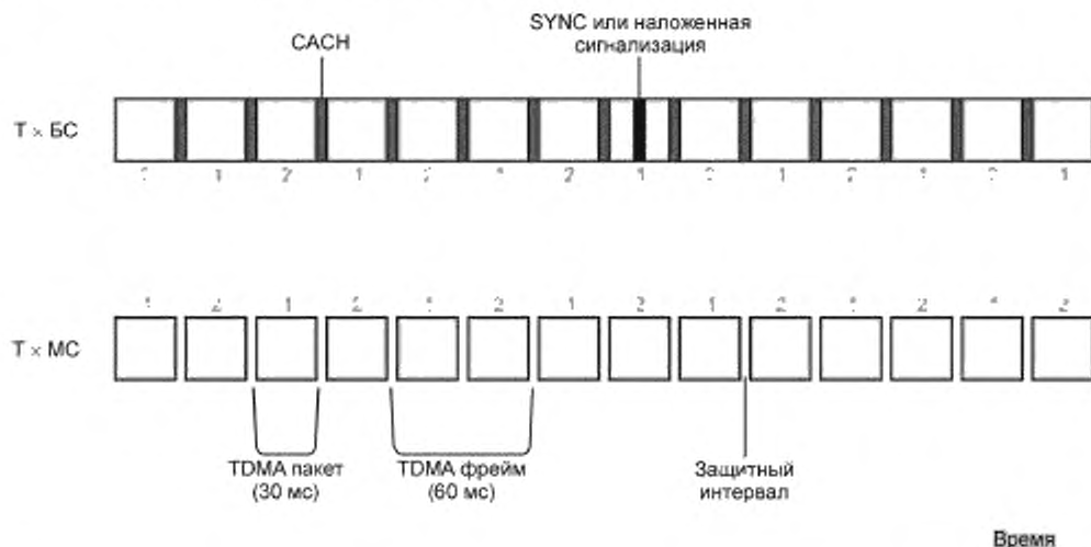
Рисунок А.2 — Диаграммы обмена между БС и МС
