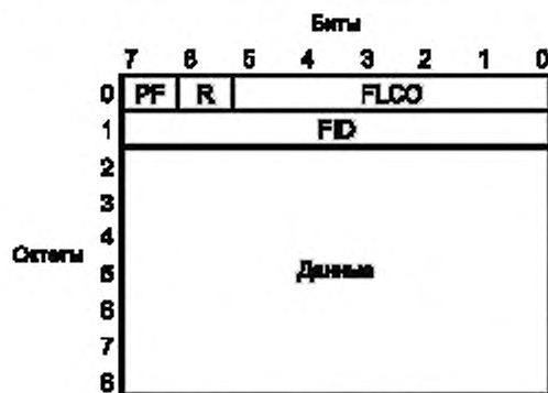
Рисунок А.20 — Общая структура полного LC сообщения
