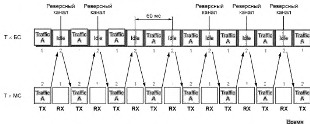
Рисунок A.15 — Синхронизация назначенного реверсивного канала
