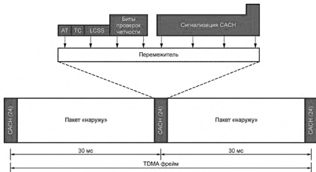
Рисунок А.17 — Формат пакета CACH
