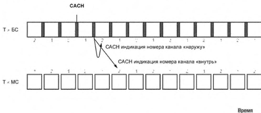
Рисунок А.8 — Синхронизация пакета CACH для индикации номера канала
