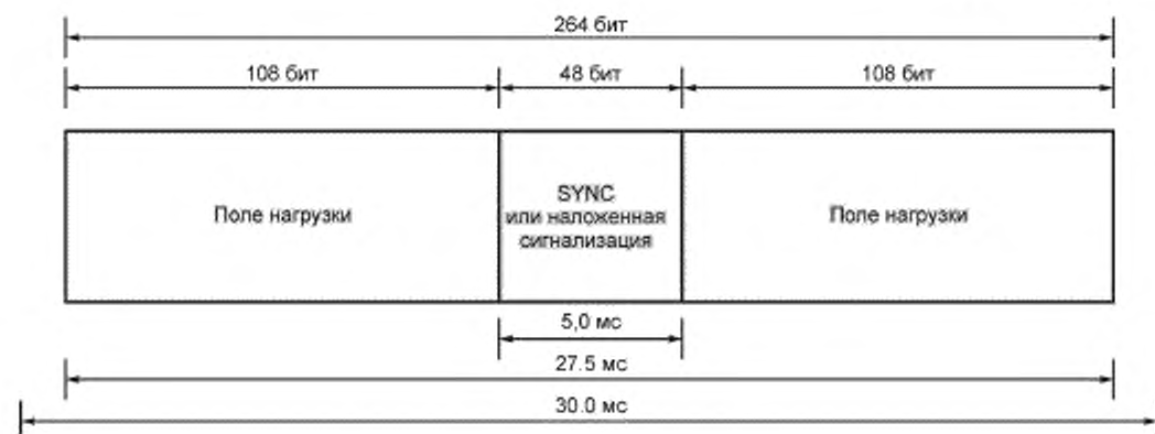
Рисунок А.3 — Общая структура пакета
