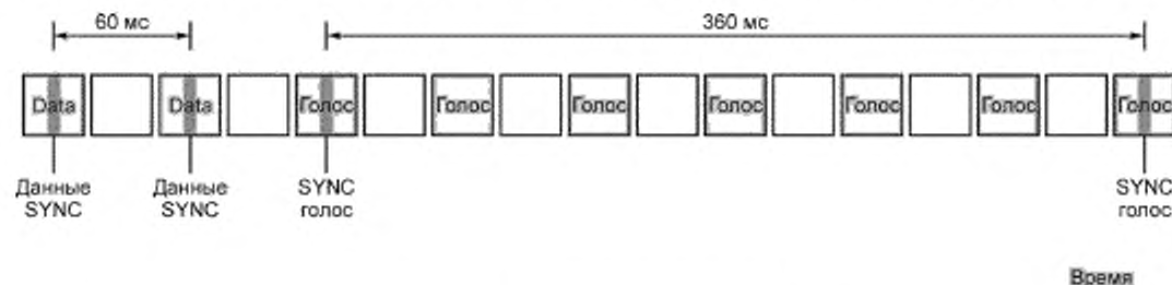
Рисунок А.6 — Синхронизация канала от МС к БС
