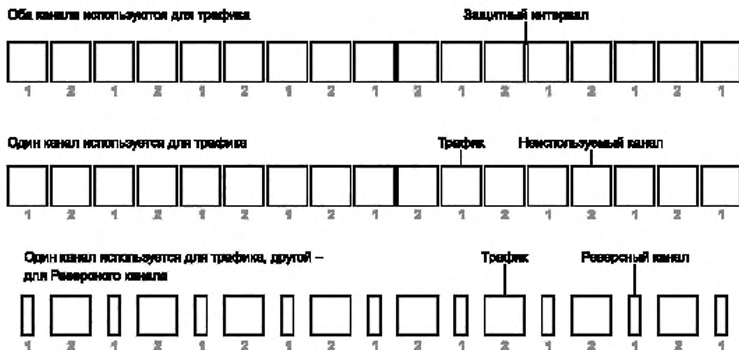
Рисунок А.9 — Канал трафика с защитным интервалом
