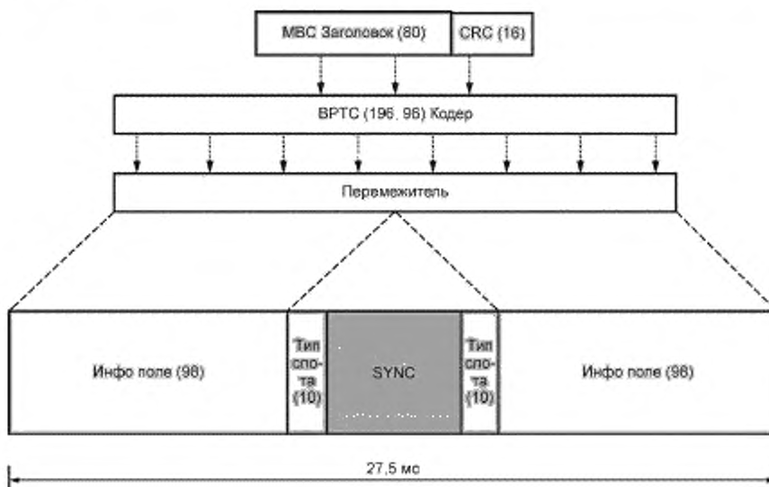
Рисунок A.26 — Формат пакета MBC заголовка сообщения
