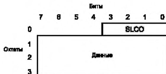
Рисунок А.21 — Структура короткого LC сообщения
