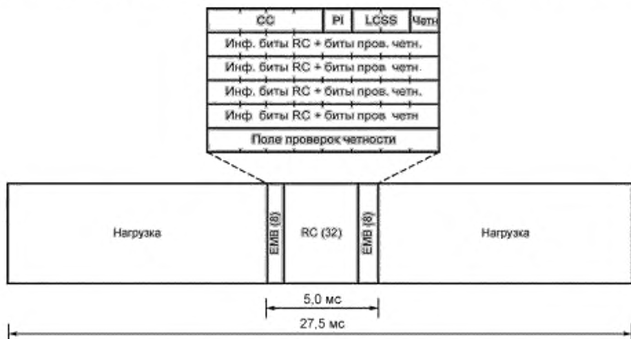
Рисунок А.19 — Формат пакета реверсного канала
