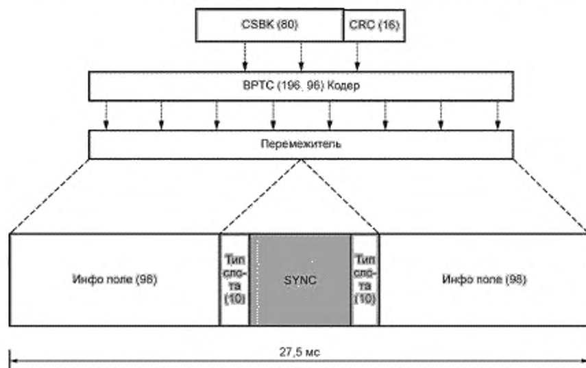
Рисунок A.25 — Формат сообщения блока управления сигнализацией (CSBK)
