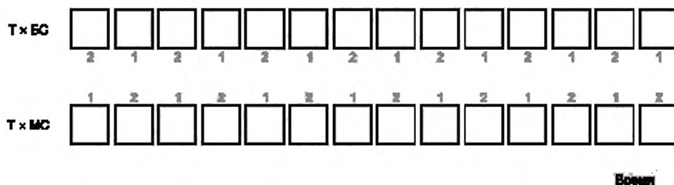
Рисунок А.14 — Синхронизация канала со сдвигом
