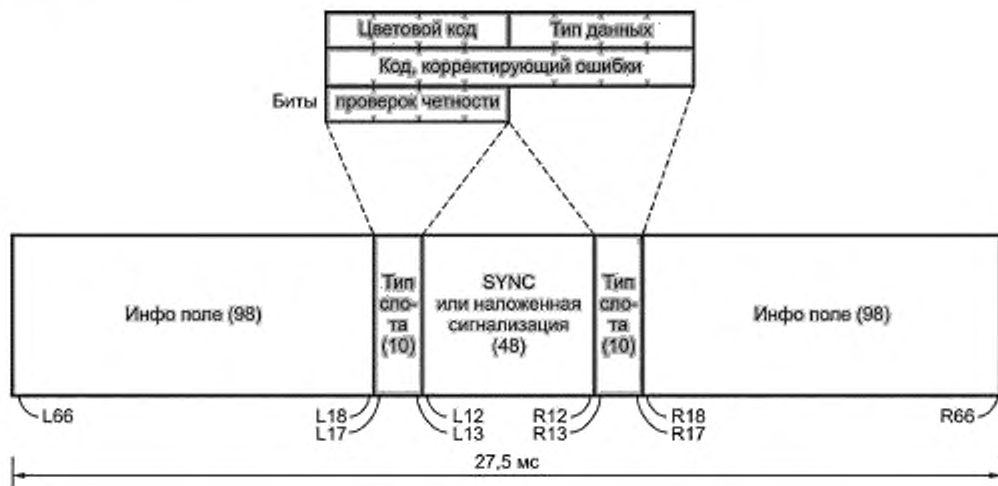
Рисунок А.16 — Формат пакета общих данных
