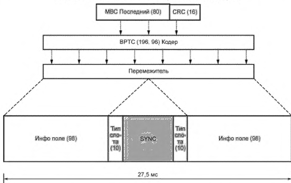
Рисунок А.28 — Формат последнего блока MBC сообщения
