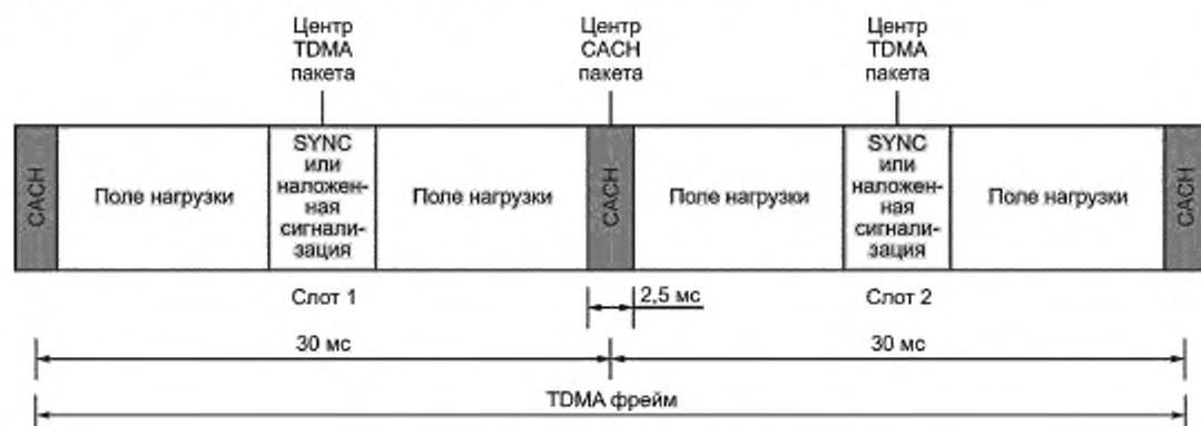
Рисунок А.5 — Структура TDMA фрейма от источника ВС
