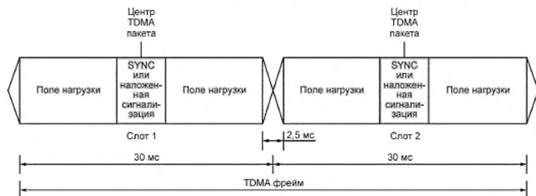
Рисунок А.4 — TDMA фрейм от источника МС
