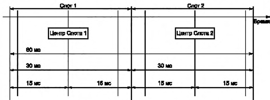
Рисунок А.12 — Синхронизация TDMA фрейма
