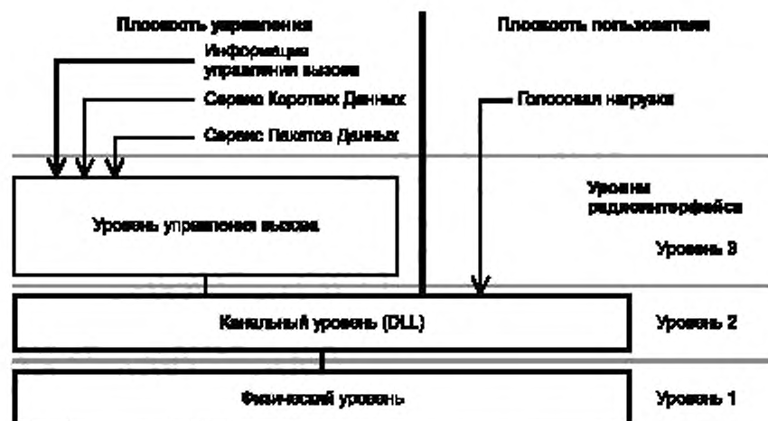
Рисунок А.1 — Стек протоколов DMR
