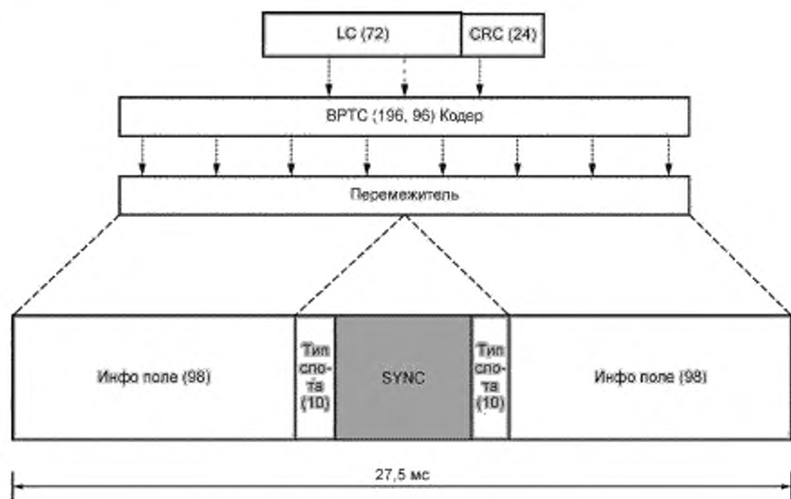
Рисунок А.23 — Формат пакета «Окончание LC»
