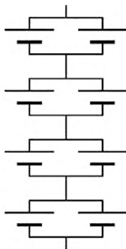
Рисунок А.4 — Структура 2P4S
