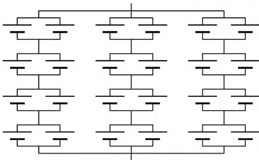
Рисунок А.5 — Структура 2P4S3P
