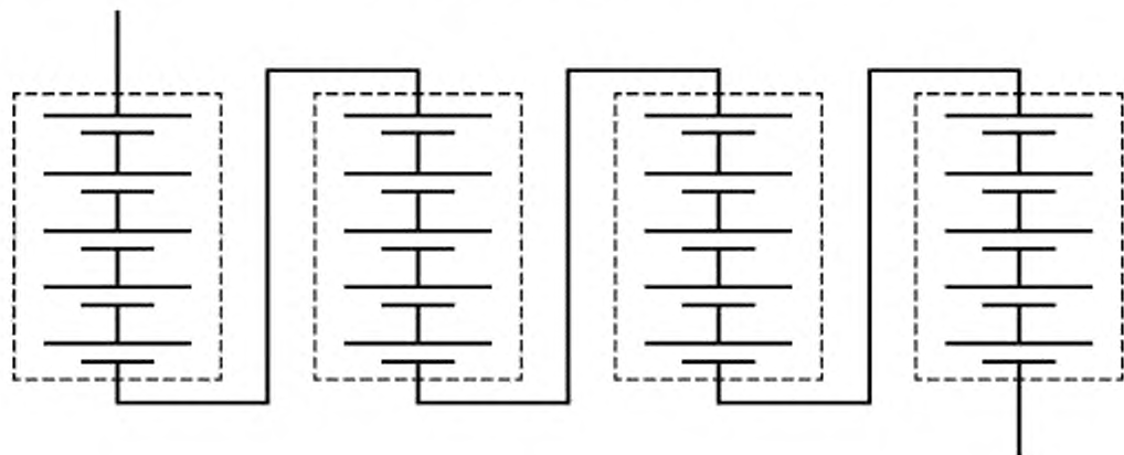
Рисунок А.8 — Структура (5S)4S
