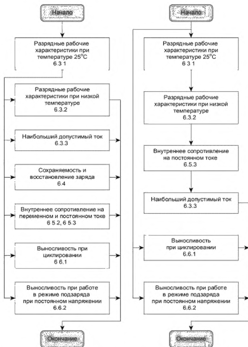
а) испытания электрических характеристик одиночных аккумуляторов и аккумуляторных блоков
