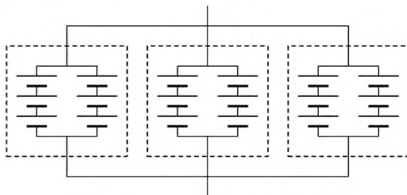
Рисунок А.7 — Структура (3S2P)3P
