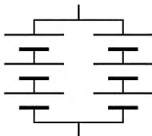
Рисунок А.3 — Структура 3S2P
