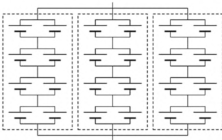
Рисунок А.6 — Структура (2P4S)3P
