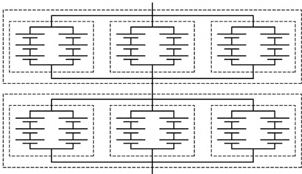
Рисунок А.9 — Структура ((3S2P)3P)2S
