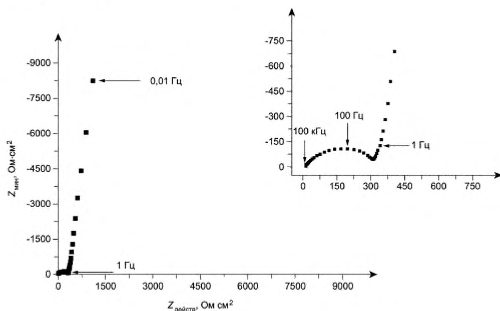
Рисунок А.4 — Годограф электрохимического импеданса
