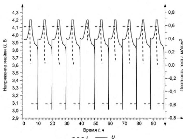
Рисунок А.5 — Циклирование в режимах по 5.4.1
