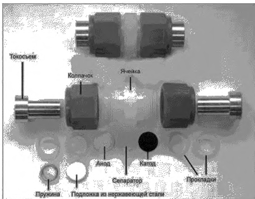
Рисунок А.1 — Отдельные части ячейки
