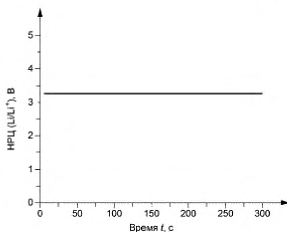
Рисунок А.3 — Зависимость НРЦ/потенциала от времени
