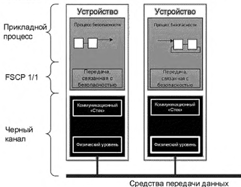
Рисунок 14 — Пример коммуникаций FSCP 1/1
