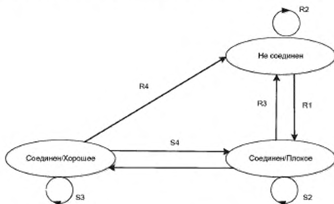
Рисунок 18 — Диаграмма перехода состояний для издателя FSCP 1/1
