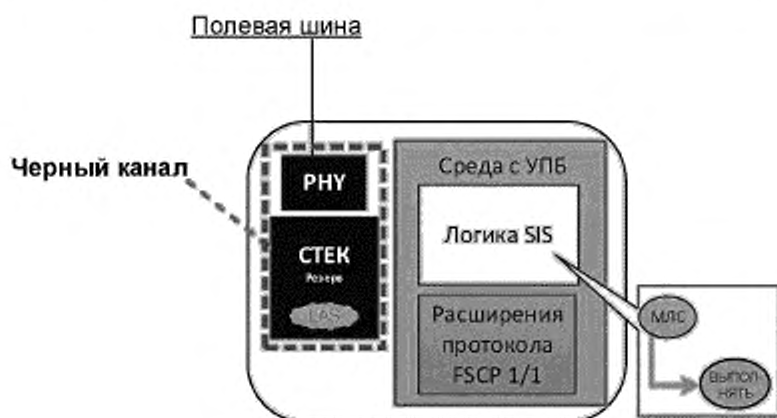
Рисунок 9 — Устройство Н1 с FSCP 1/1
