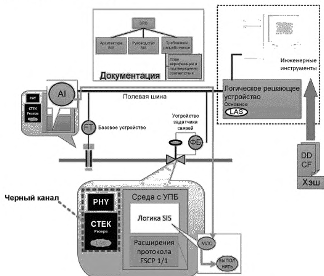
Рисунок 6 — Архитектура (H1) FSCP 1/1
