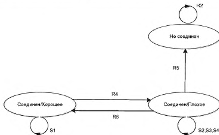
Рисунок 21 — Диаграмма перехода состояний для подписчика FSCP 1/1
