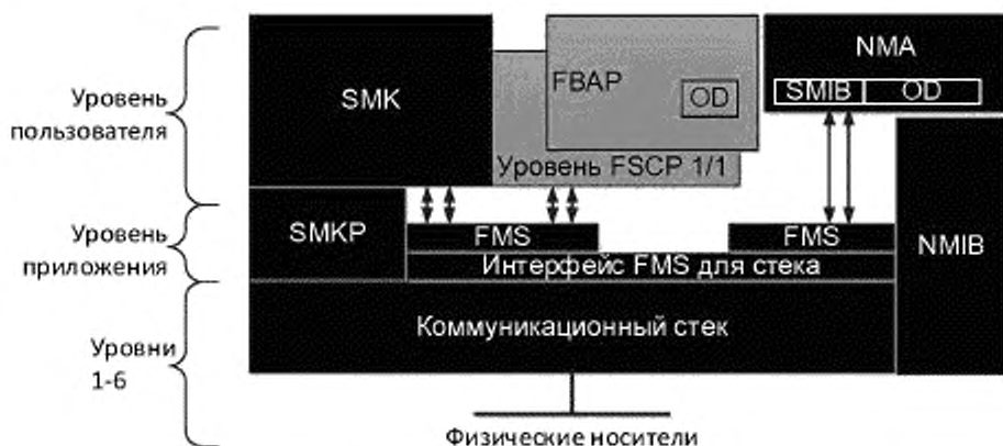
Рисунок 10 — Уровни протокола FSCP 1/1
