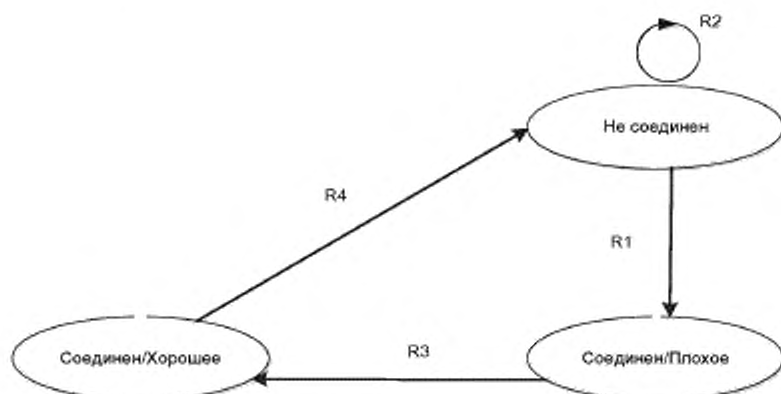
Рисунок 3 — Пример диаграммы состояний
