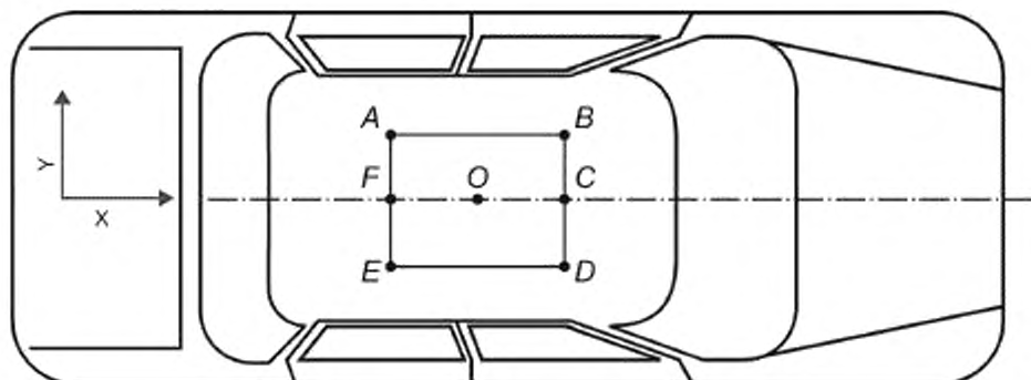
O — точка центра масс транспортного средства, расстояния OF и OC должны быть не более 70 мм, расстояния AF, BC, CD и EF должны быть не более 40 мм
