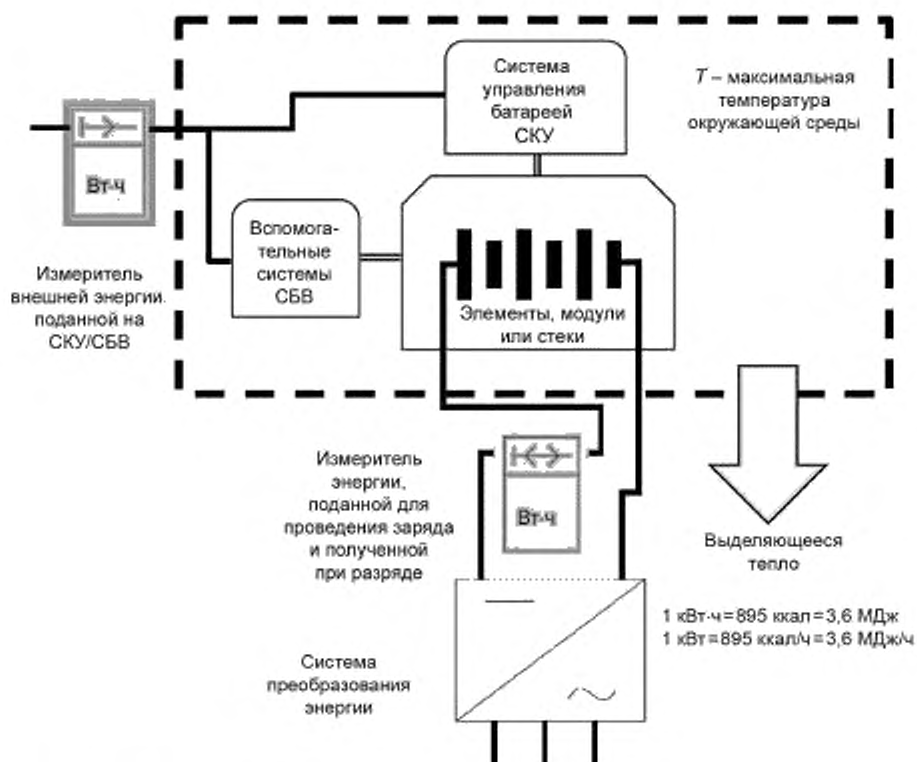
Рисунок 17 — Схематическое представление расположения двух точек измерения энергии (энергии к вспомогательным системам и энергии к и от батареи), используемых для определения энергии, выделяющейся и отводимой в виде тепла
