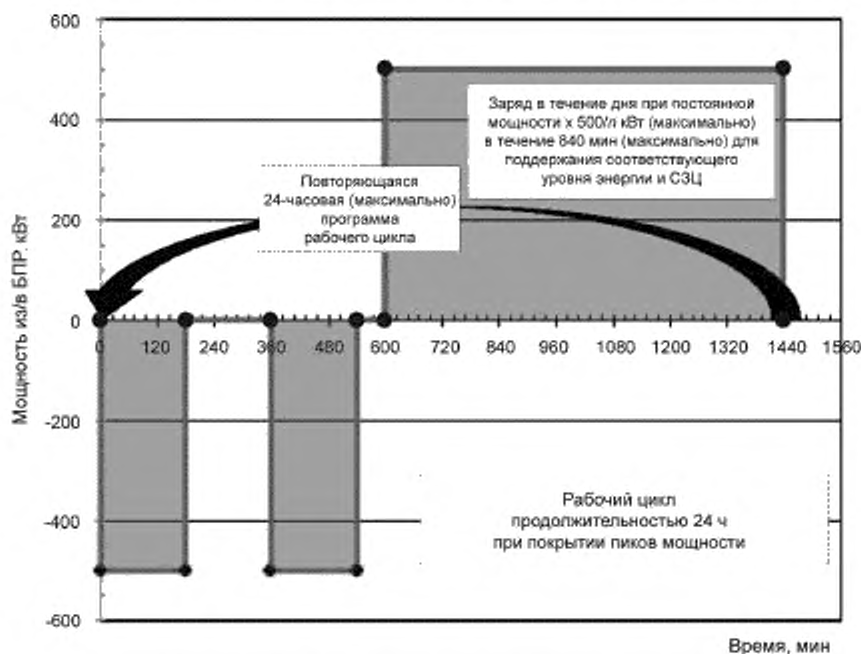
Рисунок 13 — Профиль программы работы в режиме покрытия дневных пиков мощности (см. 6.4)
